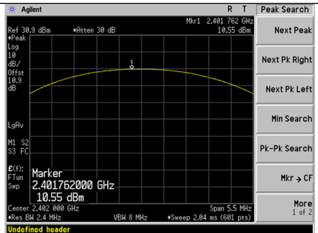
OUTPUT POWER \pi/4 -DQPSK low
