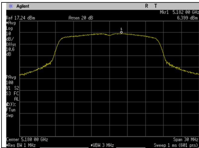
U-NII-1_5180MHz_Low Ch_36_20MHz BW_a-mode_Spectral Density
