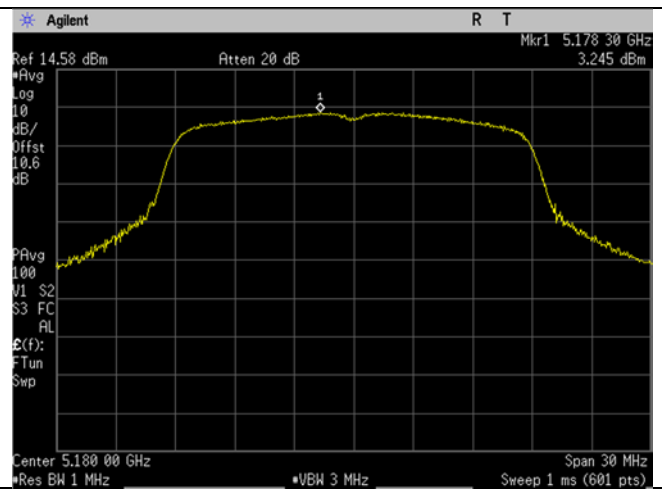
U-NII-1_5180MHz_Low Ch_36_20MHz BW_n/ac-mode_Spectral Density
