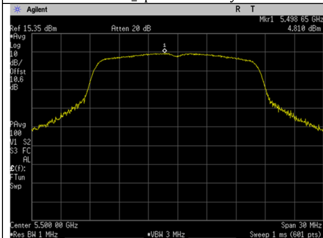
U-NII-2C_5500MHz_Low Ch_100_20MHz BW_a-mode_Spectral Density
