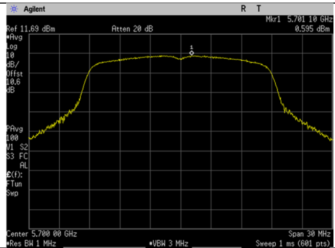
U-NII-2C_5700MHz_High Ch_140_20MHz BW_n/ac-mode_Spectral Density
