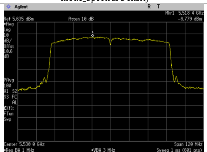
U-NII-2C_5530MHz_Low Ch_106_80MHz BW_n/ac-mode_Spectral Density
