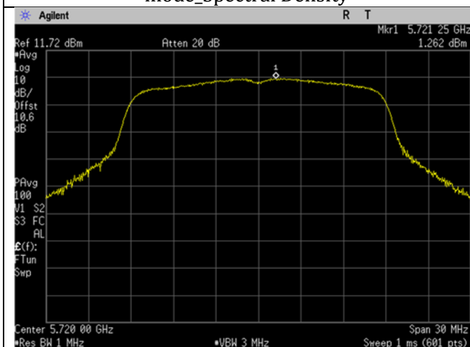
U-NII-2C_5720MHz_High Ch_144_20MHz BW_n/ac-mode_Spectral Density
