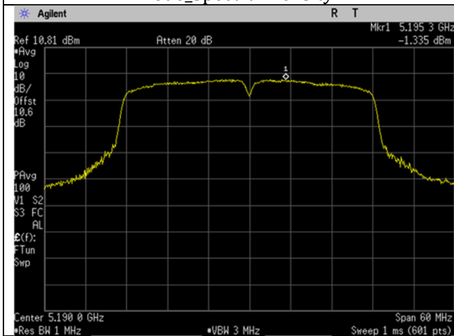
U-NII-1_5190MHz_Low Ch_38_40MHz BW_n/ac-mode_Spectral Density
