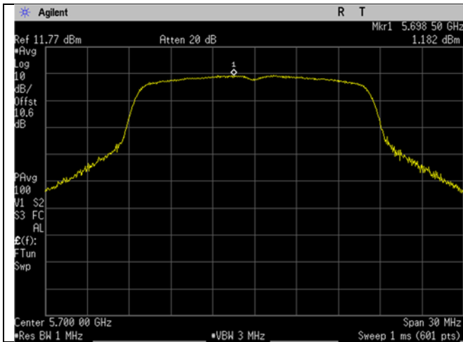
U-NII-2C_5700MHz_High Ch_140_20MHz BW_a-mode_Spectral Density
