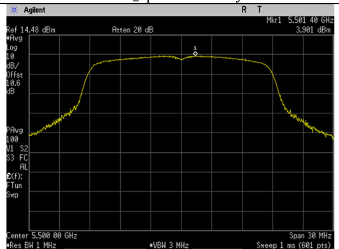
U-NII-2C_5500MHz_Low Ch_100_20MHz BW_n/ac-mode_Spectral Density
