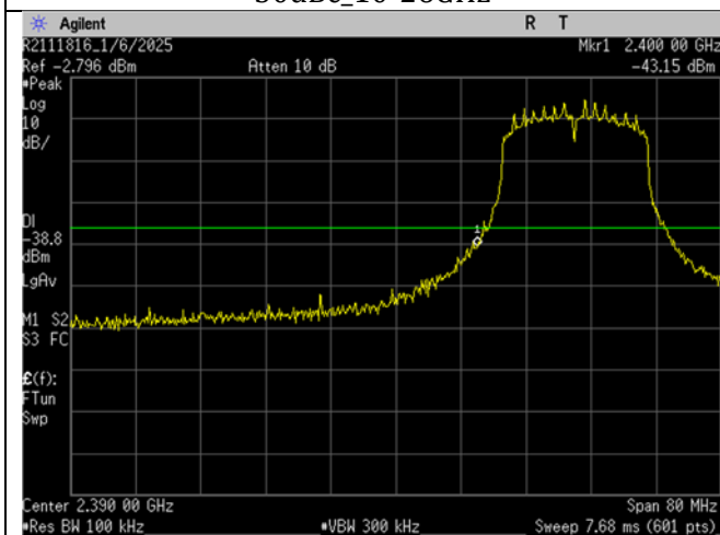
WIFI_Low Ch_2412MHz_20MHz BW_n-mode_- 30dBc_Lower Band Edge
