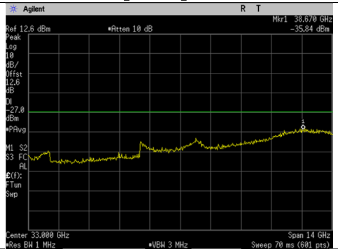
U-NII-2C_5600MHz_Mid Ch_120_20MHz BW_n/ac-mode_-27dBm_26-40GHz
