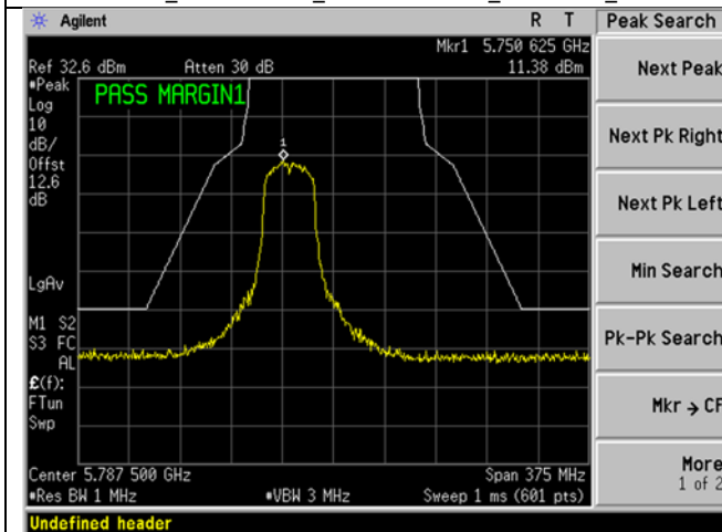
U-NII-3_5755MHz_40MHz BW_n/ac-mode_Mask
