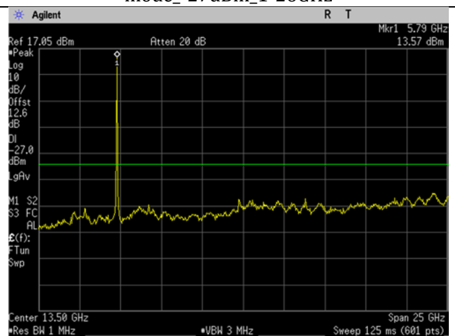
U-NII-3_5785MHz_Mid Ch_157_20MHz BW_n/ac- mode_-27dBm_1-26GHz
