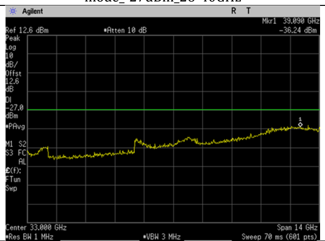
U-NII-2C_5610MHz_Mid Ch_122_80MHz BW_ac-mode_-27dBm_26-40GHz
