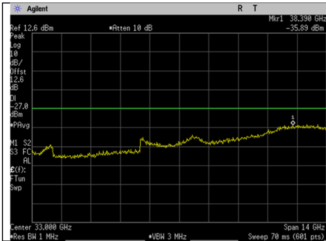
U-NII-1_5180MHz_Low Ch_36_20MHz BW_n/ac-mode_-27dBm_26-40GHz
