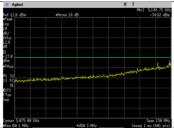
U-NII-1_5180MHz_Low Ch_36_20MHz BW_n/ac-mode_-27dBm_Lower Band Edge
