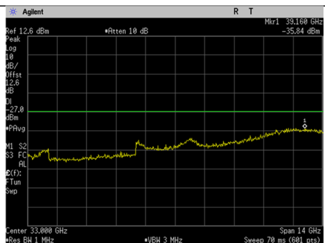
U-NII-1_5180MHz_Low Ch_36_20MHz BW_a-mode_-27dBm_26-40GHz
