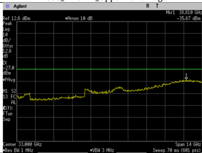
U-NII-2C_5690MHz_High Ch_138_80MHz BW_ac-mode_-27dBm_26-40GHz
