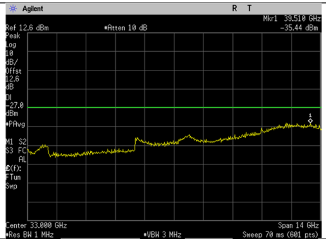
U-NII-2A_5260MHz_low_mid Ch_52_20MHz BW_a-mode_-27dBm_26-40GHz
