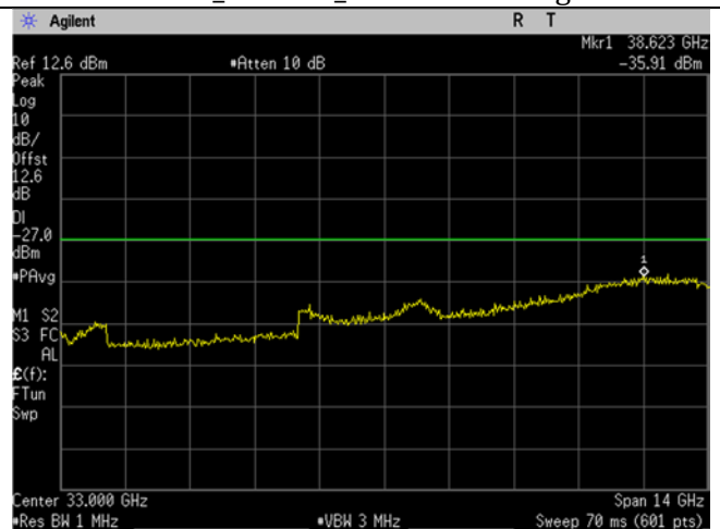
U-NII-1_5190MHz_Low Ch_38_40MHz BW_n/ac-mode_-27dBm_26-40GHz
