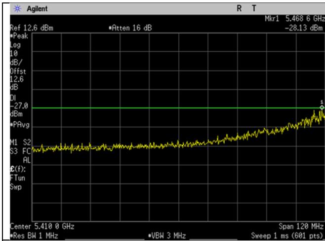
U-NII-2C_5510MHz_Low Ch_102_40MHz BW_n/ac-mode_-27dBm_Lower Band Edge
