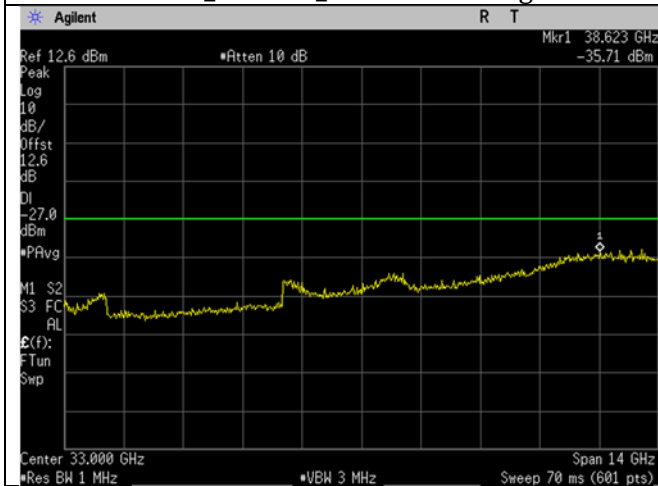
U-NII-2C_5530MHz_Low Ch_106_80MHz BW_ac-mode_-27dBm_26-40GHz
