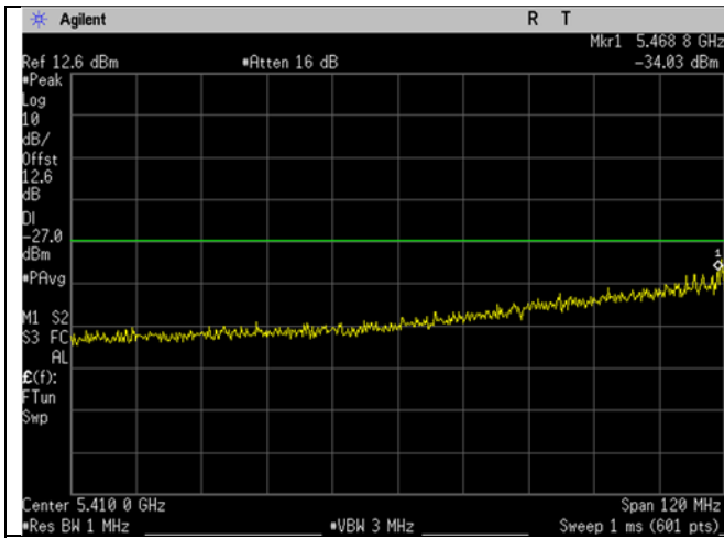
U-NII-2C_5500MHz_Low Ch_100_20MHz BW_a-mode_-27dBm_Lower Band Edge
