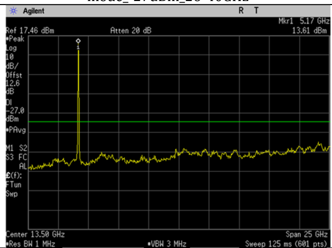
U-NII-1_5180MHz_Low Ch_36_20MHz BW_n/ac-mode_-27dBm_1-26GHz
