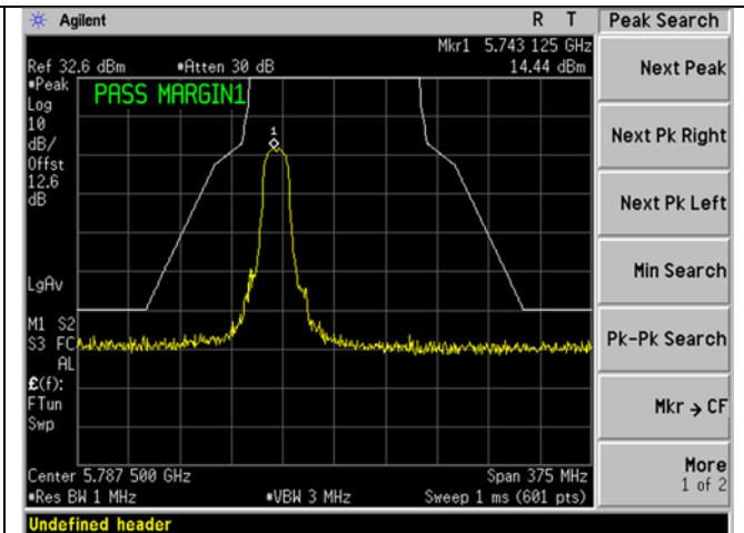
U-NII-3_5745MHz_20MHz BW_n/ac-mode_Mask
