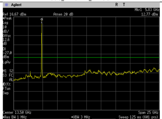
U-NII-3_5825MHz_High Ch_165_20MHz BW_n/ac-mode_-27dBm_1-26GHz
