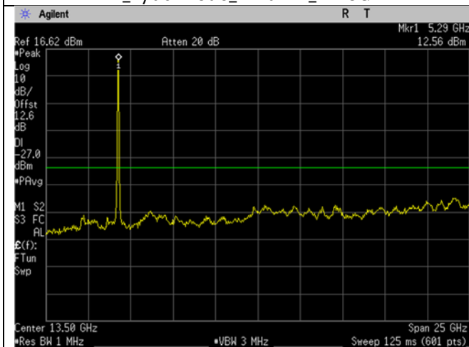
U-NII-2A_5270MHz_low_Mid Ch_54_40MHz BW_n/ac-mode_-27dBm_1-26GHz
