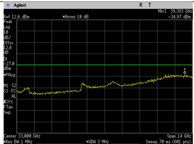
U-NII-2C_5700MHz_High Ch_140_20MHz BW_a-mode_-27dBm_26-40GHz
