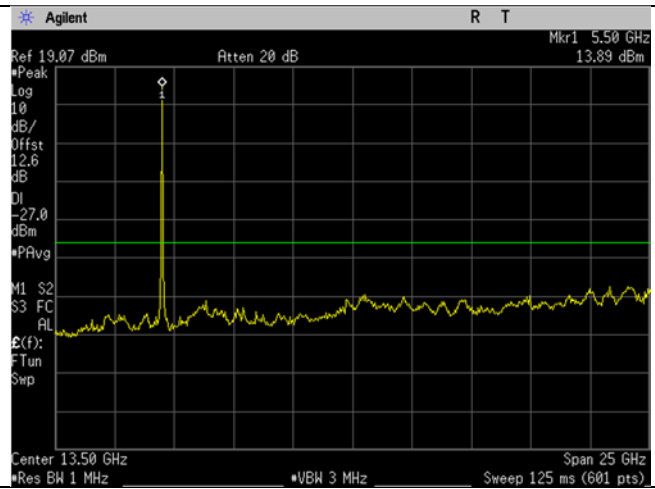
U-NII-2C_5500MHz_Low Ch_100_20MHz BW_n/ac-mode_-27dBm_1-26GHz
