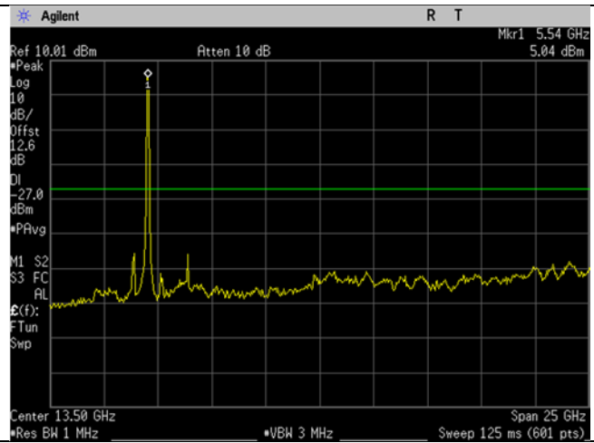
U-NII-2C_5530MHz_Low Ch_106_80MHz BW_ac-mode_-27dBm_1-26GHz
