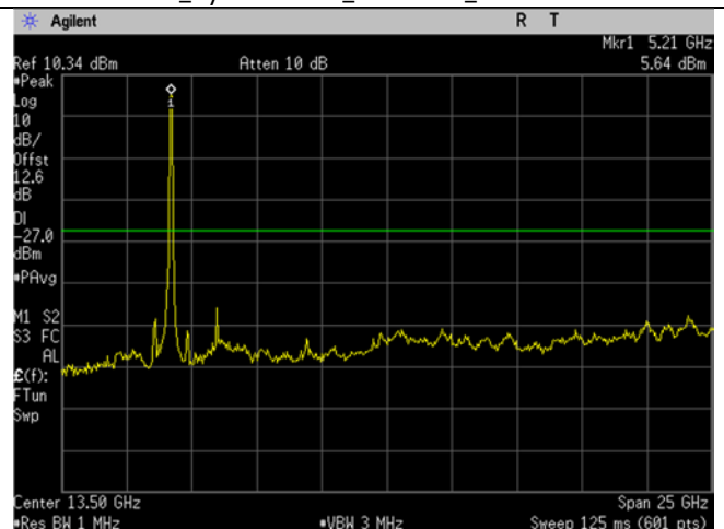
U-NII-1_5210MHz_Low Mid Ch_42_80MHz BW_ac- mode_-27dBm_1-26GHz
