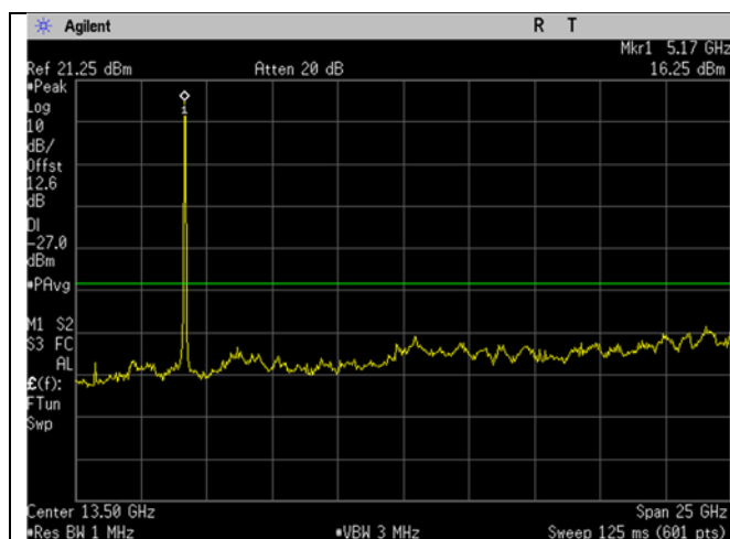
U-NII-1_5180MHz_Low Ch_36_20MHz BW_a-mode_-27dBm_1-26GHz
