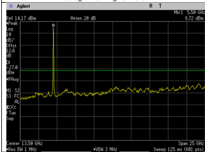
U-NII-2C_5510MHz_Low Ch_102_40MHz BW_n/ac-mode_-27dBm_1-26GHz
