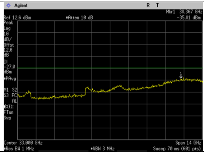
U-NII-2C_5670MHz_High Ch_134_40MHz BW_n/ac-mode_-27dBm_26-40GHz
