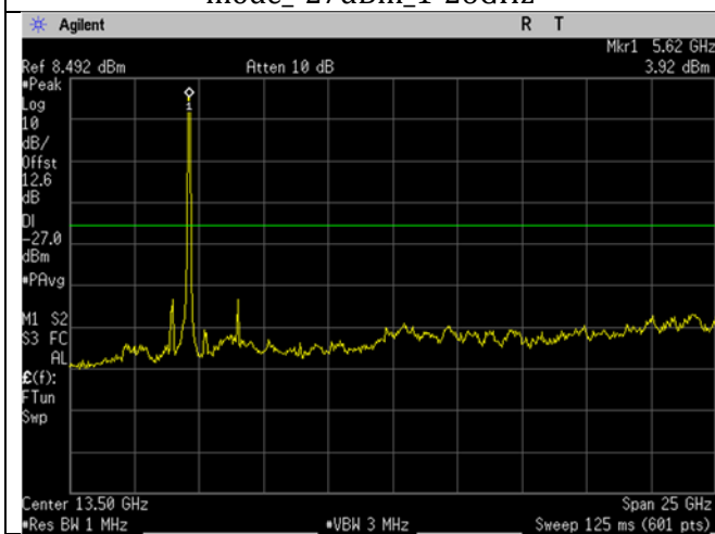
U-NII-2C_5610MHz_Mid Ch_122_80MHz BW_ac-mode_-27dBm_1-26GHz
