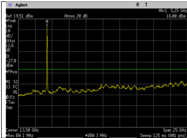
U-NII-2A_5260MHz_low_mid Ch_52_20MHz BW_a-mode_-27dBm_1-26GHz
