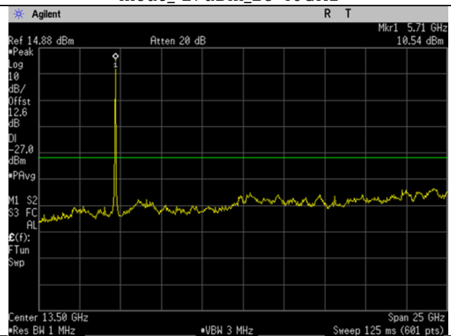
U-NII-2C_5700MHz_High Ch_140_20MHz BW_n/ac-mode_-27dBm_1-26GHz
