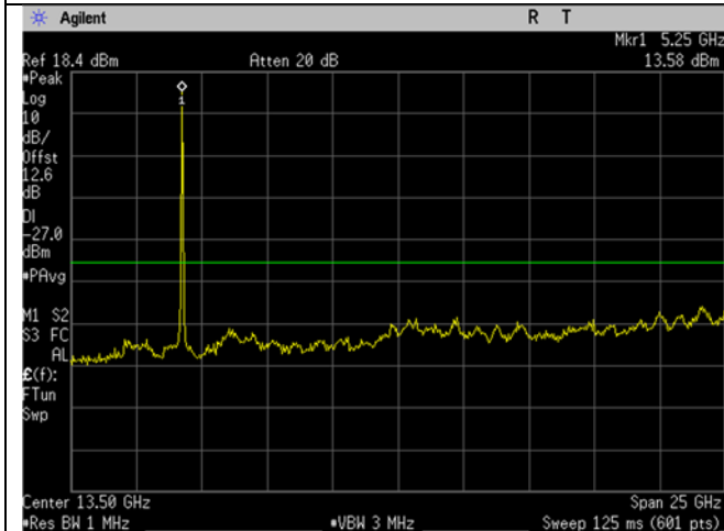
U-NII-2A_5260MHz_low_mid Ch_52_20MHz BW_n/ac-mode_-27dBm_1-26GHz
