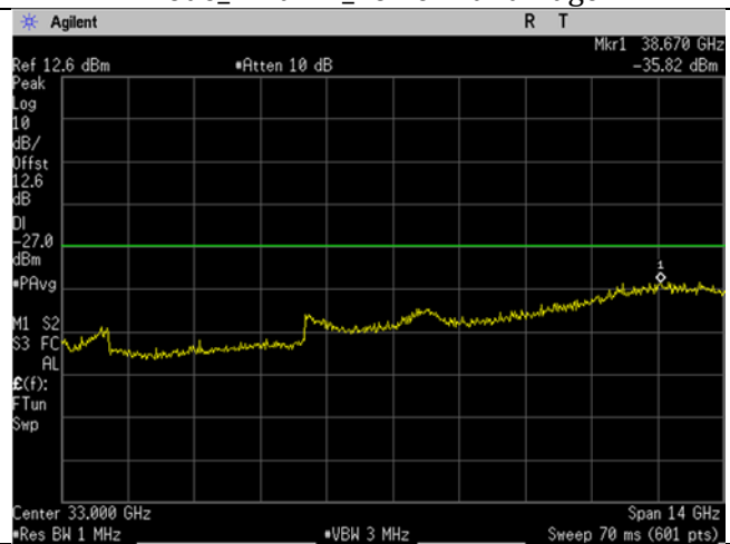
U-NII-2C_5510MHz_Low Ch_102_40MHz BW_n/ac-mode_-27dBm_26-40GHz
