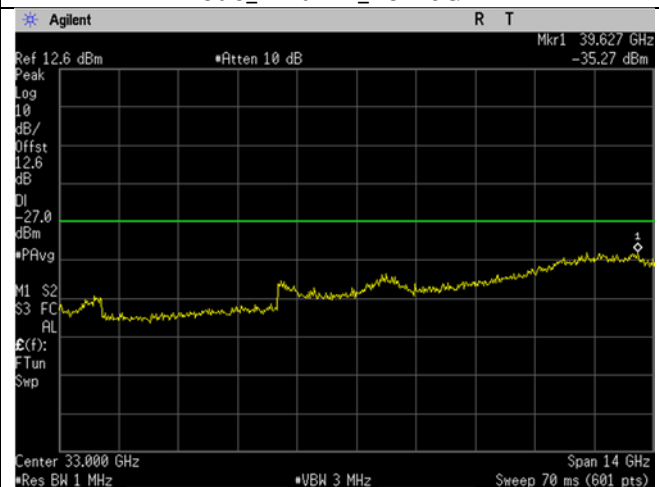
U-NII-2C_5720MHz_High Ch_144_20MHz BW_n/ac-mode_-27dBm_26-40GHz
