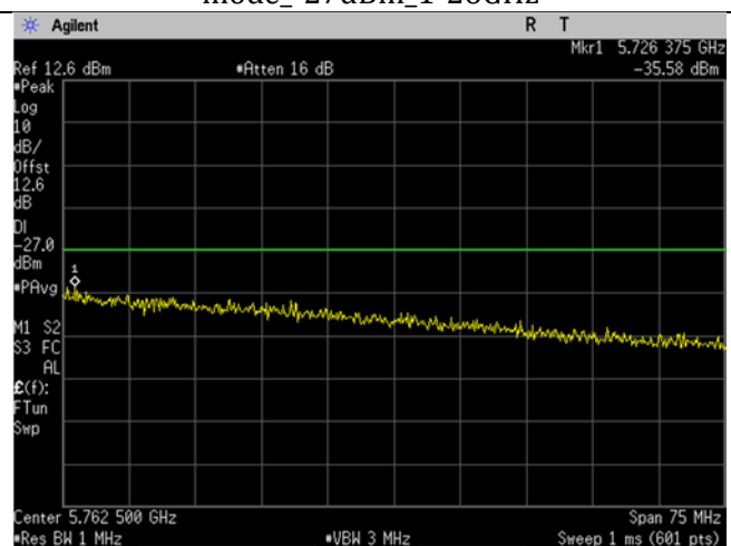
U-NII-2C_5700MHz_High Ch_140_20MHz BW_n/ac-mode_-27dBm_Upper Band Edge
