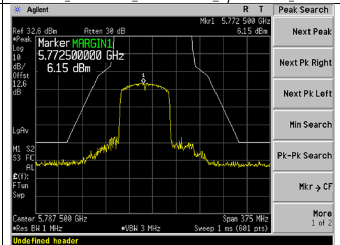
U-NII-3_5775MHz_80MHz BW_ac-mode_Mask
