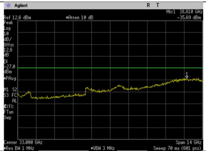
U-NII-1_5230MHz_high_Mid Ch_46_40MHz BW_n/ac-mode_-27dBm_26-40GHz
