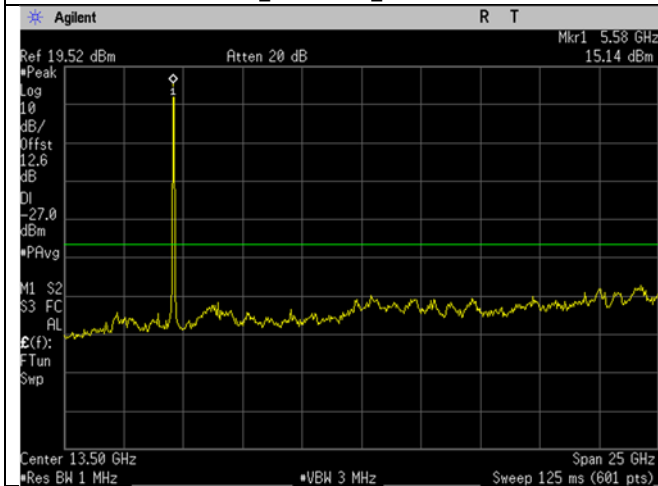
U-NII-2C_5600MHz_Mid Ch_120_20MHz BW_n/ac-mode_-27dBm_1-26GHz
