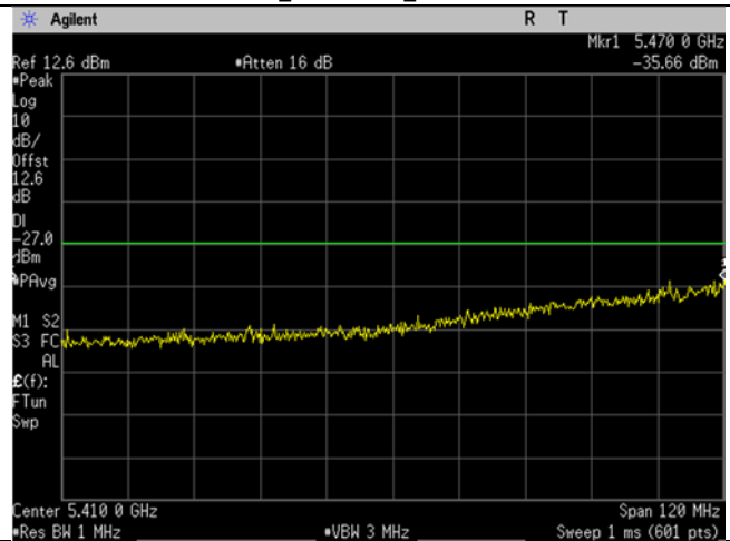
U-NII-2C_5500MHz_Low Ch_100_20MHz BW_n/ac-mode_-27dBm_Lower Band Edge
