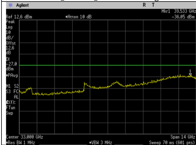
U-NII-2C_5500MHz_Low Ch_100_20MHz BW_n/ac-mode_-27dBm_26-40GHz
