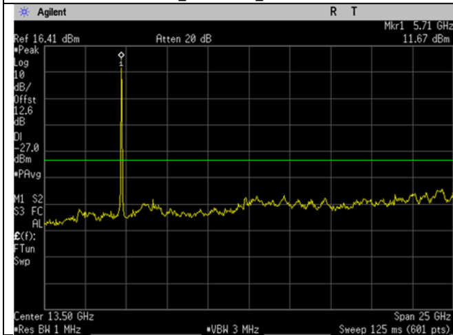
U-NII-2C_5720MHz_High Ch_144_20MHz BW_a-mode_-27dBm_1-26GHz
