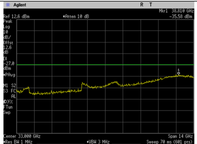
U-NII-2A_5260MHz_low_mid Ch_52_20MHz BW_n/ac-mode_-27dBm_26-40GHz
