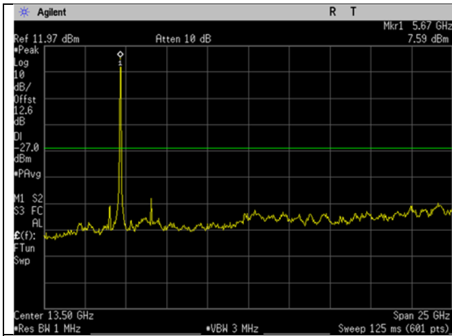
U-NII-2C_5670MHz_High Ch_134_40MHz BW_n/ac-mode_-27dBm_1-26GHz
