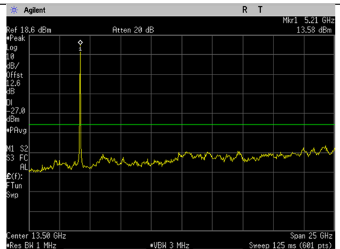
U-NII-1_5200MHz_low_Mid Ch_40_20MHz BW_n/ac-mode_-27dBm_1-26GHz
