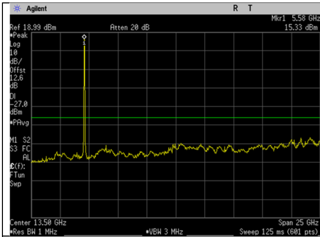
U-NII-2C_5600MHz_Mid Ch_120_20MHz BW_a-mode_-27dBm_1-26GHz
