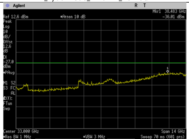
U-NII-2A_5270MHz_low_Mid Ch_54_40MHz BW_n/ac-mode_-27dBm_26-40GHz
