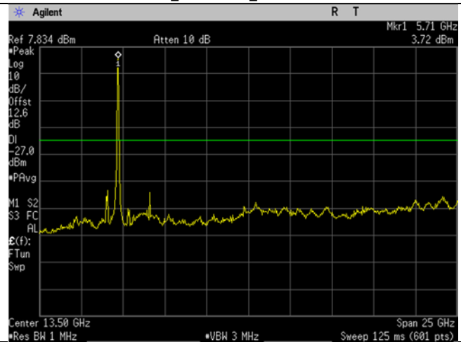
U-NII-2C_5690MHz_High Ch_138_80MHz BW_ac-mode_-27dBm_1-26GHz
