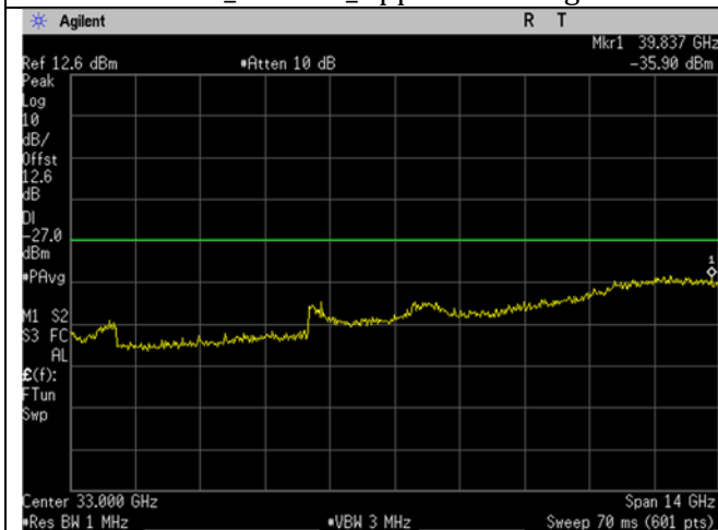
U-NII-2A_5320MHz_High Ch_64_20MHz BW_n/ac-mode_-27dBm_26-40GHz
