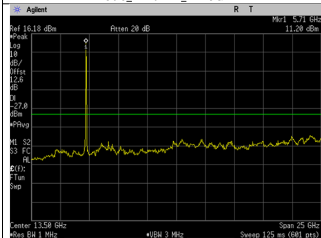
U-NII-2C_5720MHz_High Ch_144_20MHz BW_n/ac-mode_-27dBm_1-26GHz
