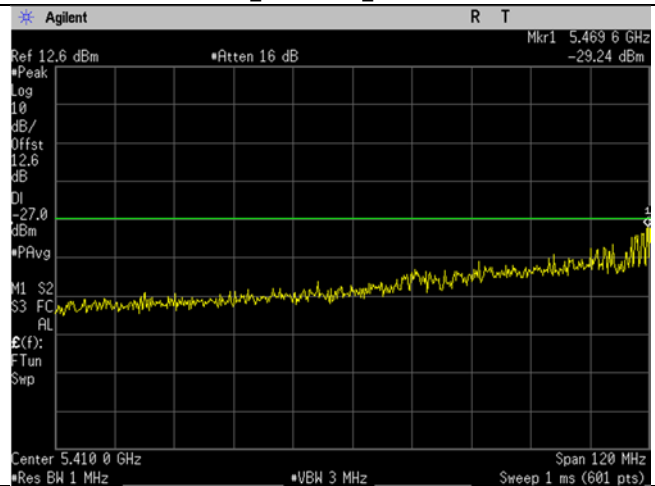
U-NII-2C_5530MHz_Low Ch_106_80MHz BW_ac-mode_-27dBm_Lower Band Edge
