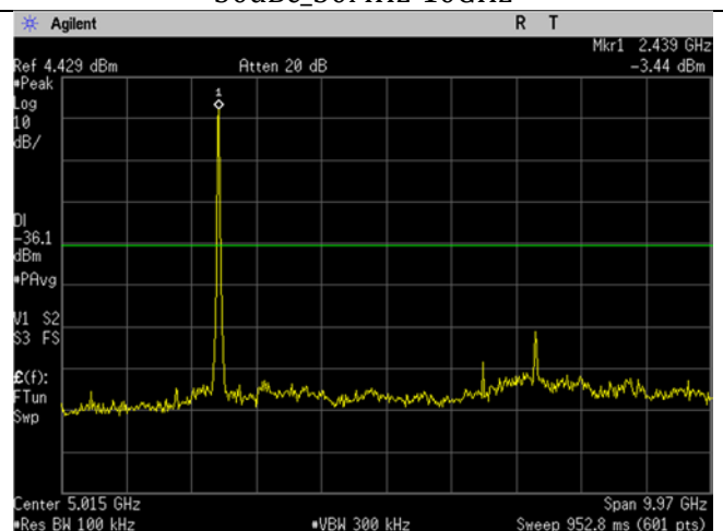
WIFI_Mid Ch_2437MHz_20MHz BW_g-mode_-30dBc_30MHz-10GHz
