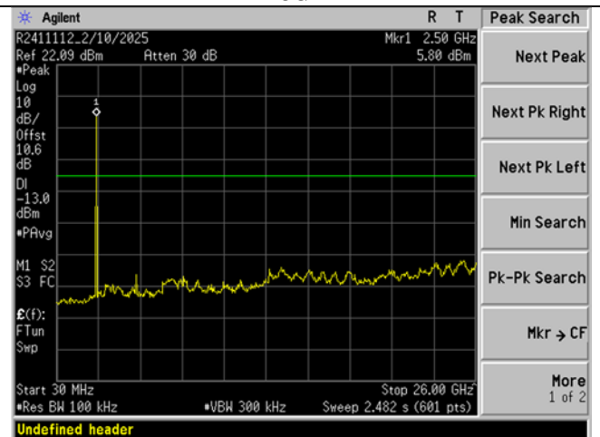
BLE_High Ch_2480MHz_2MBit_-20dBc_30MHz- 26GHz
