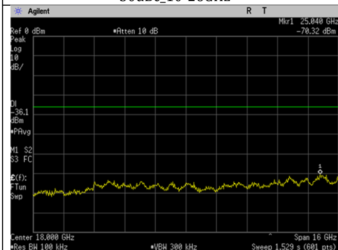
WIFI_Mid Ch_2437MHz_20MHz BW_g-mode_-30dBc_10-26GHz
