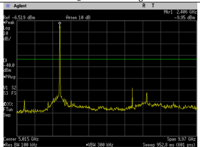
WIFI_Low Ch_2412MHz_20MHz BW_g-mode_-30dBc_30MHz-10GHz
