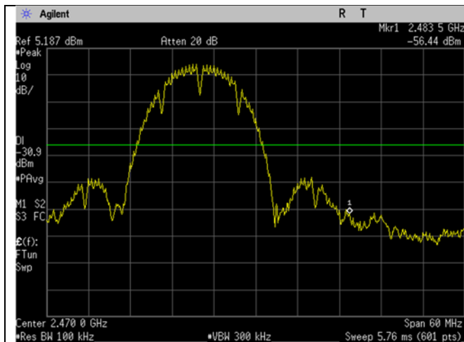
WIFI_High Ch_2462MHz_20MHz BW_b-mode_-20dBc_Upper Band Edge
