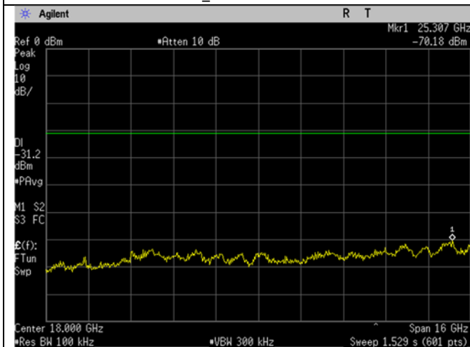
WIFI_Mid Ch_2437MHz_20MHz BW_b-mode_-30dBc_10-26GHz
