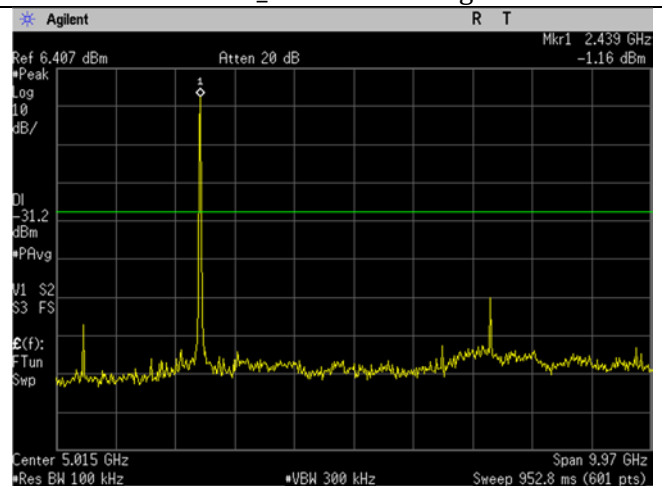
WIFI_Mid Ch_2437MHz_20MHz BW_b-mode_-30dBc_30MHz-10GHz
