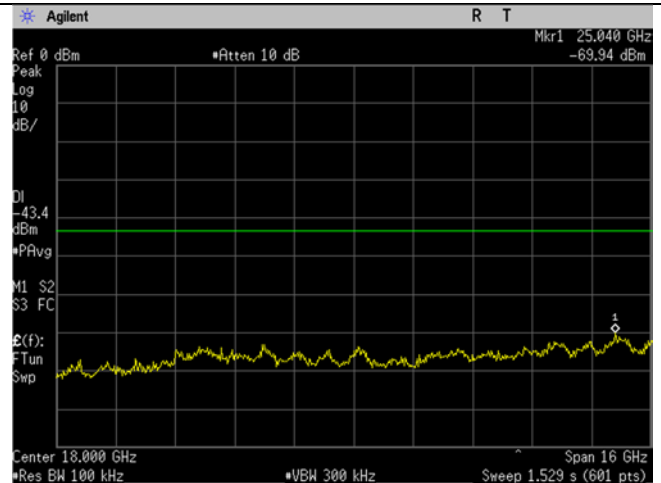
WIFI_High Ch_2462MHz_20MHz BW_n-mode_- 30dBc_10-26GHz
