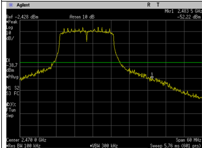
WIFI_High Ch_2462MHz_20MHz BW_n-mode_- 20dBc_Upper Band Edge
