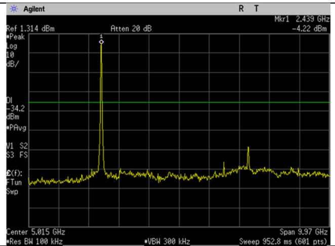
WIFI_Mid Ch_2437MHz_20MHz BW_n-mode_- 30dBc_30MHz-10GHz
