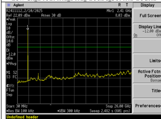
Low Ch_2402MHz_2DH1_-20dBc_30MHz-26GHz
