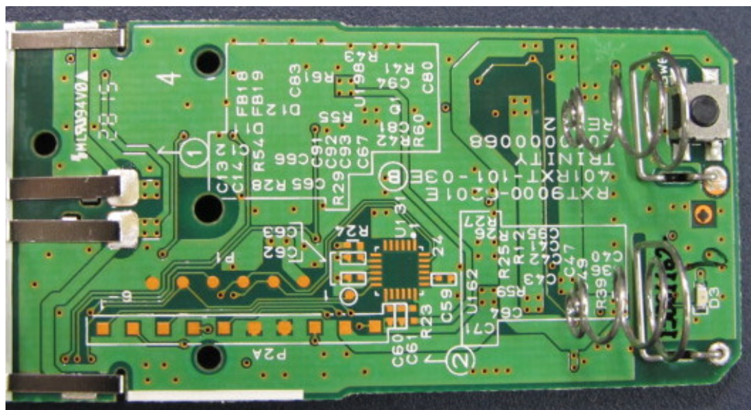
Antenna RF IC ATMEL OZMO2000 Antenna Crystal OSC 24MHz(Y1)
