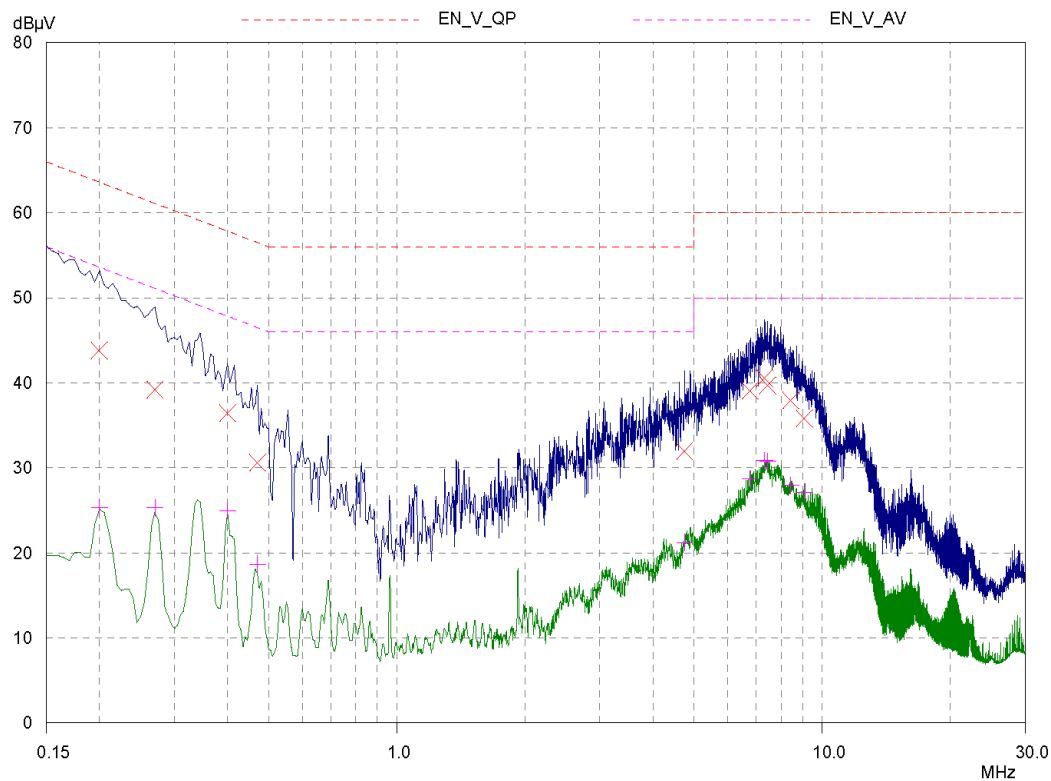
Neutral – PE
