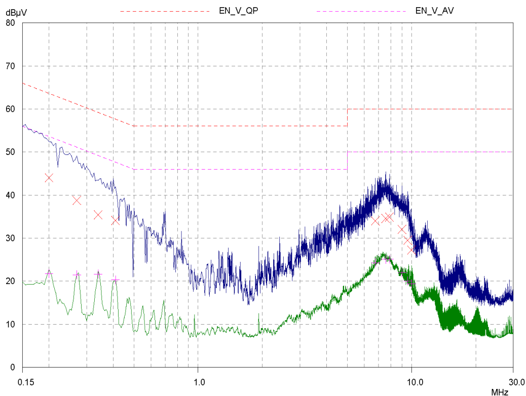
Neutral – PE
