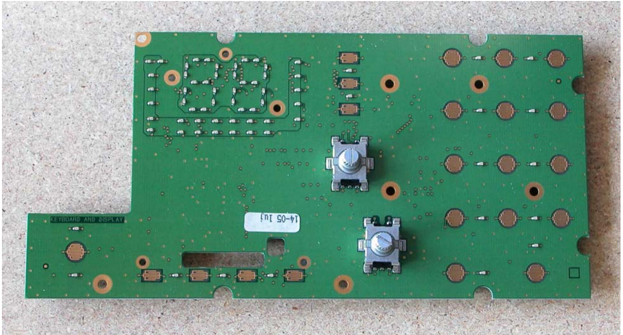
Keyboard / Display module 639130, upper layer
