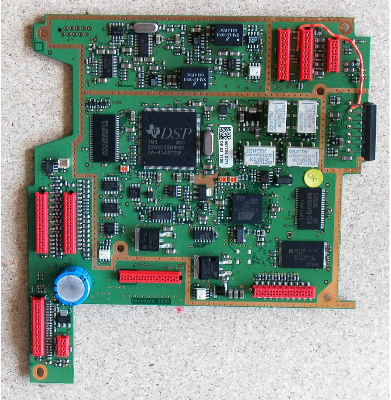
Base Band module 639110, upper layer
