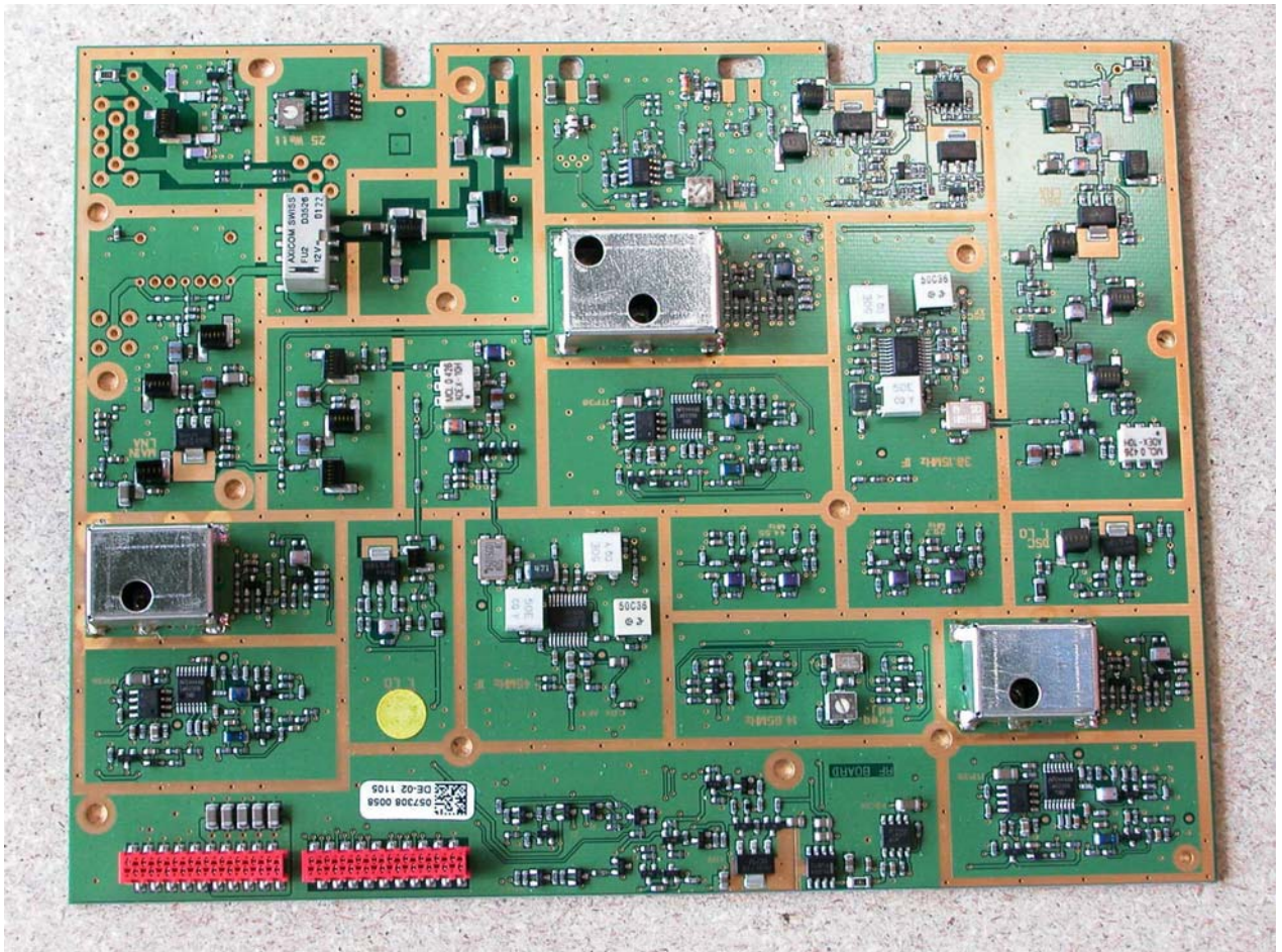
RF module 639120, upper layer
