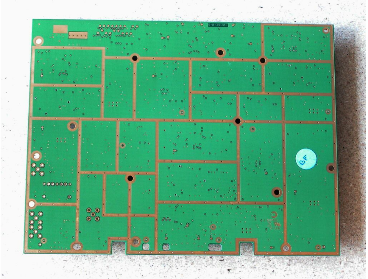
RF module 639120, lower layer
