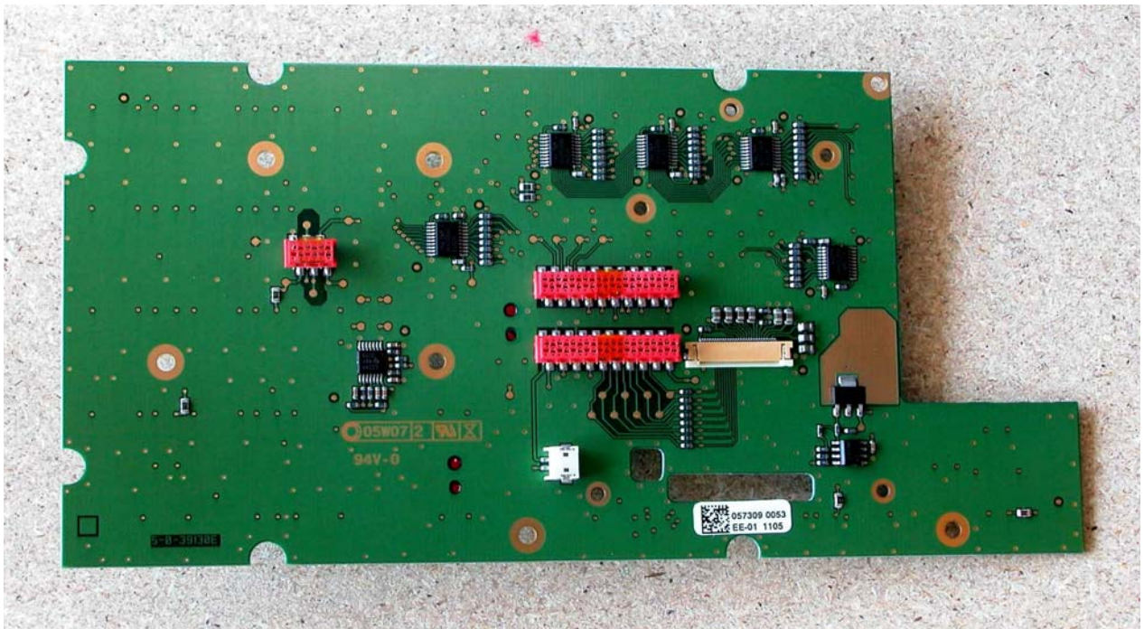
Keyboard / Display module 639130, lower layer
