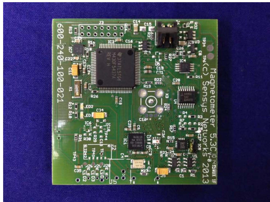
(4) EUT Photo
