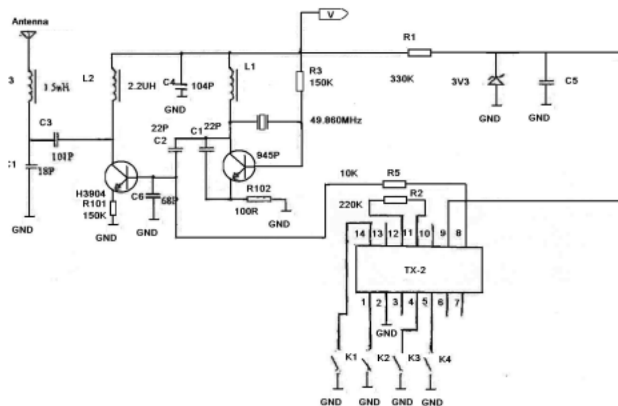
凯利达ZN-428F原理图
