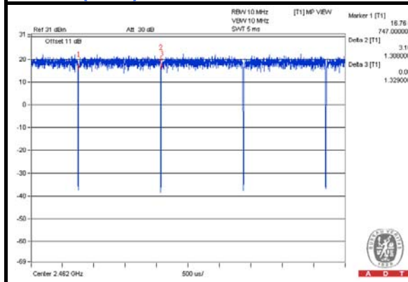
802.11n (HT20)
