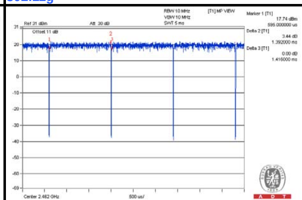
802.11n (HT40)
