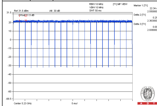
802.11n (40MHz)
