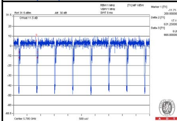
802.11n (HT40)
