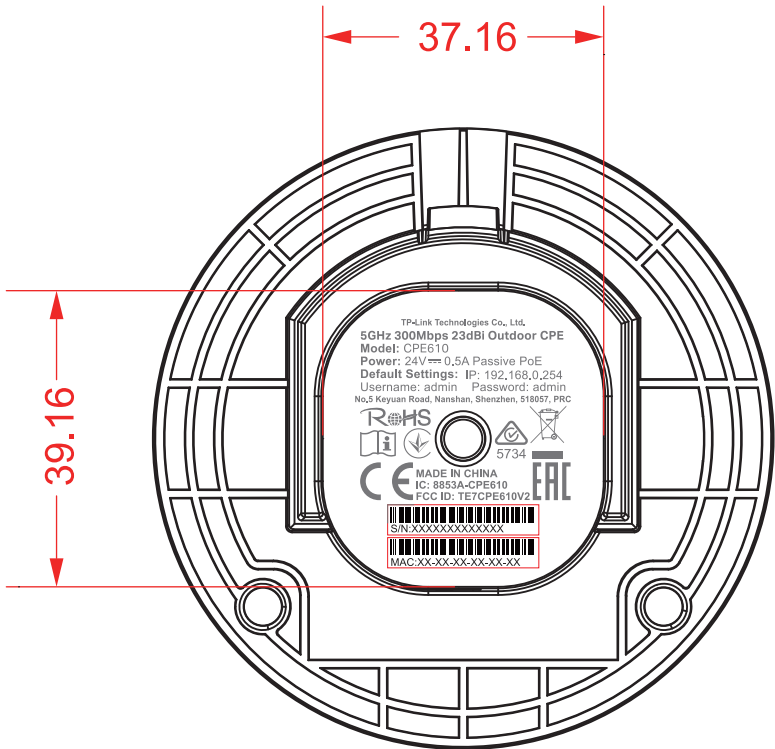
尺寸圖
