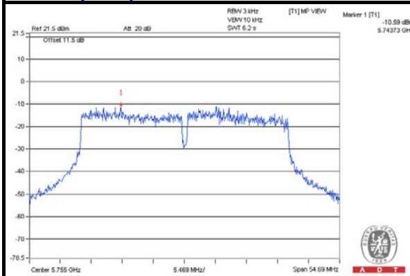
802.11n (HT40)
