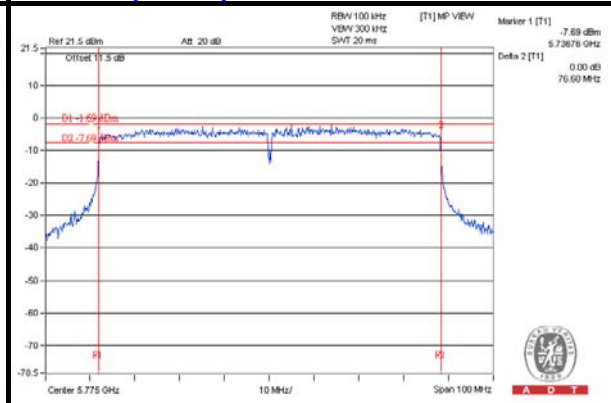
802.11ac (VHT80)
