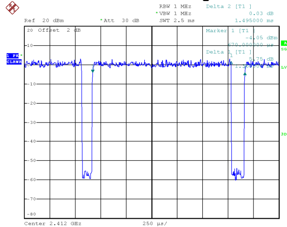
IEEE 802.11g
