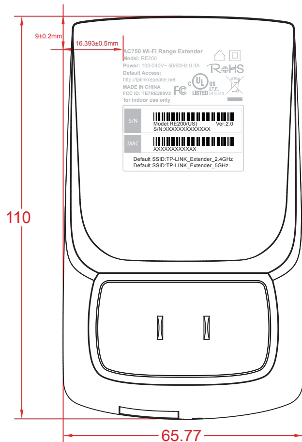
尺寸图
