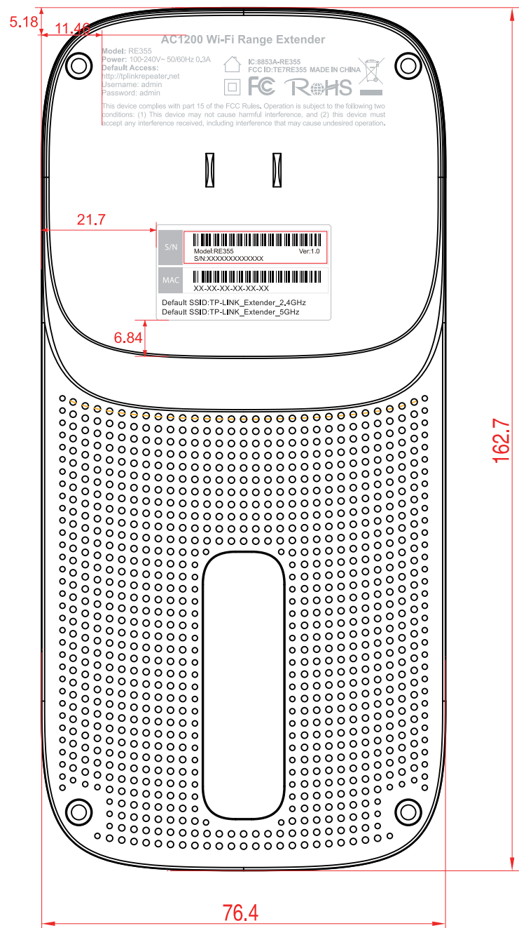
尺寸图 (标贴为粘贴)
