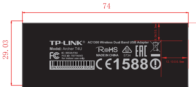
尺寸效果图
