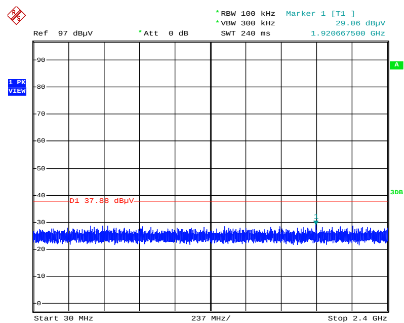
Plot on Configuration IEEE 802.11b / CH 1 / 30MHz~2400MHz (down 30dBc)
