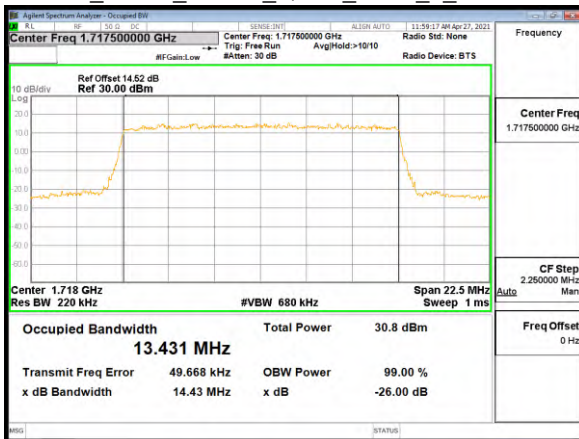
OBW_Band4_15MHz_QPSK_RB75_0_CH20175
