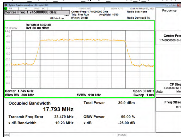
OBW_Band4_20MHz_QPSK_RB100_0_CH20300
