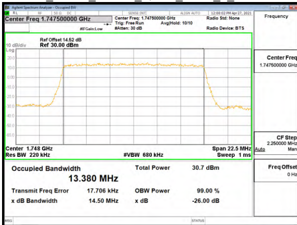
OBW_Band4_15MHz_QPSK_RB75_0_CH20325
