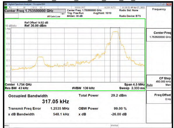
OBW_Band4_3MHz_16QAM_RB1_14_CH20385
