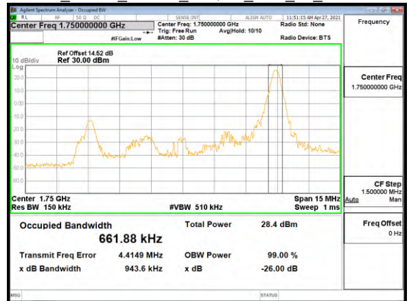
OBW_Band4_10MHz_16QAM_RB1_49_CH20350
