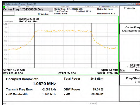
OBW_Band4_1.4MHz_QPSK_RB6_0_CH20393
