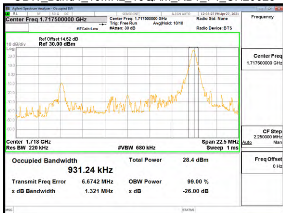
OBW_Band4_15MHz_16QAM_RB1_74_CH20175
