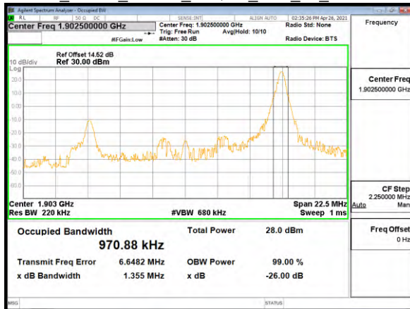
OBW_Band2_15MHz_16QAM_RB1_74_CH19125
