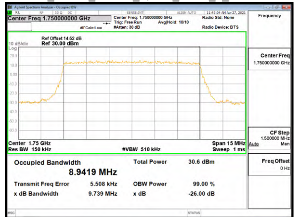
OBW_Band4_10MHz_QPSK_RB50_0_CH20350
