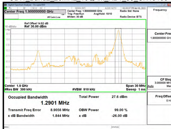
OBW_Band2_20MHz_16QAM_RB1_99_CH19100
