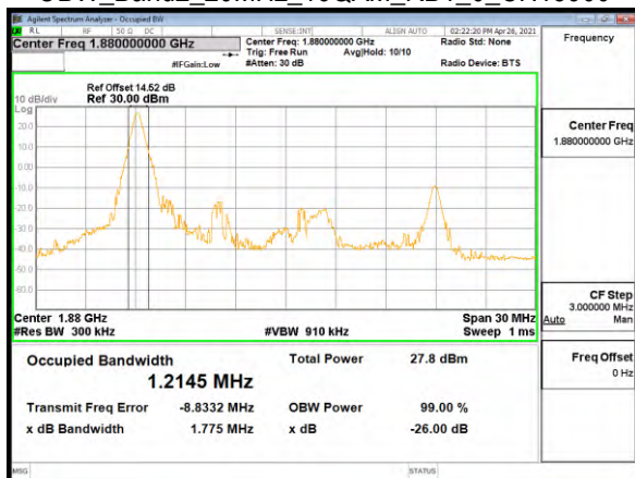
OBW_Band2_20MHz_16QAM_RB1_0_CH19100
