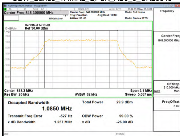
OBW_Band5_1.4MHz_QPSK_RB6_0_CH20643
