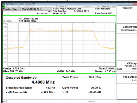
OBW_Band4_5MHz_QPSK_RB25_0_CH20375
