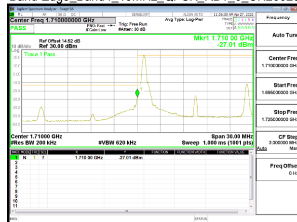
Band Edge_Band4_15MHz_QPSK_RB1_74_CH20325
