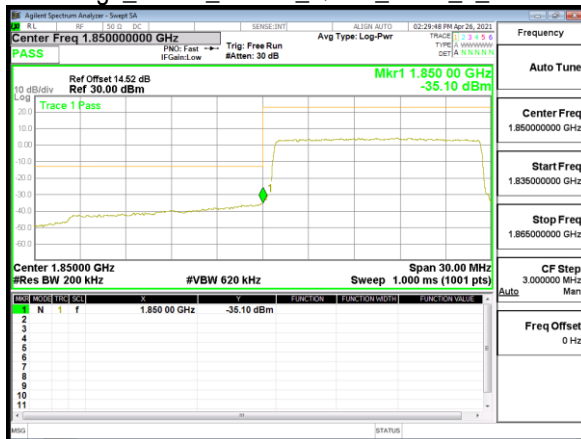
Band Edge_Band2_15MHz_QPSK_RB75_0_CH19125
