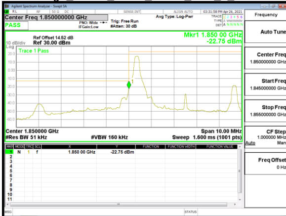
Band Edge_Band2_5MHz_QPSK_RB1_0_CH18625
