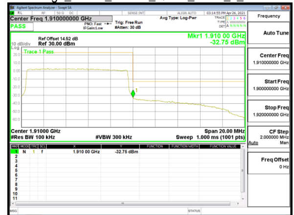
Band Edge_Band2_15MHz_QPSK_RB1_0_CH18675
