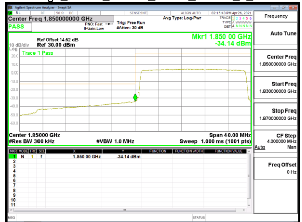
Band Edge_Band2_20MHz_QPSK_RB100_0_CH19100
