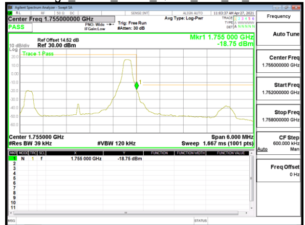
Band Edge_Band4_3MHz_QPSK_RB1_14_CH20385
