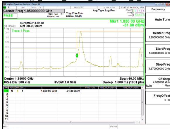
Band Edge_Band2_20MHz_QPSK_RB1_0_CH18700
