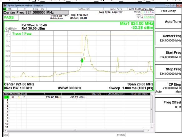
Band Edge_Band5_10MHz_QPSK_RB1_49_CH20600
