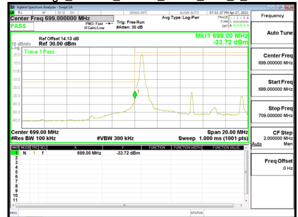
Band Edge_Band12_10MHz_QPSK_RB1_49_CH23130
