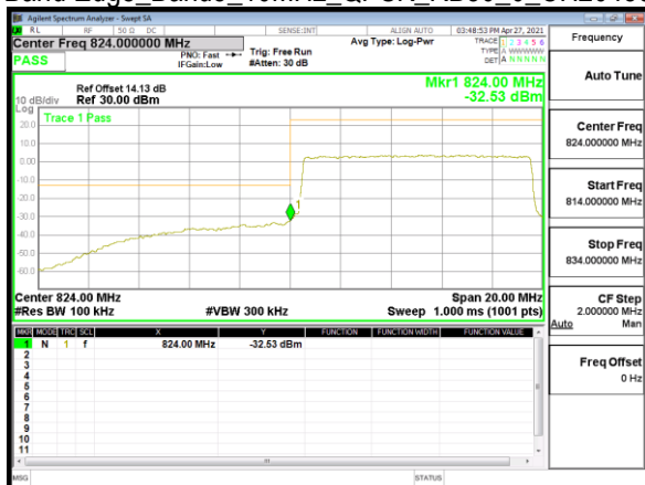
Band Edge_Band5_10MHz_QPSK_RB50_0_CH20450
