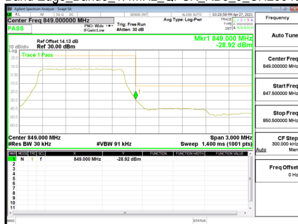
Band Edge_Band5_3MHz_QPSK_RB1_0_CH20415
