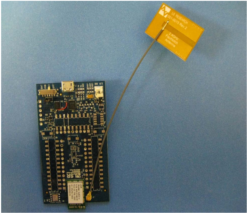
FlexNotch Antenna
