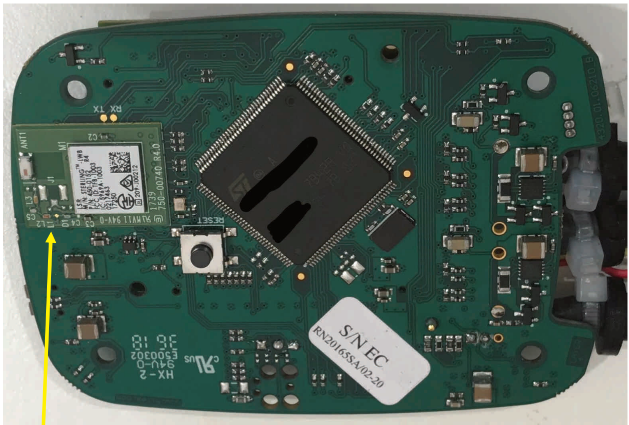
Laird 450-015 module
