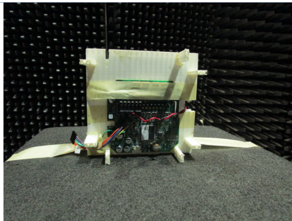
EUT Horizontal Orientation
