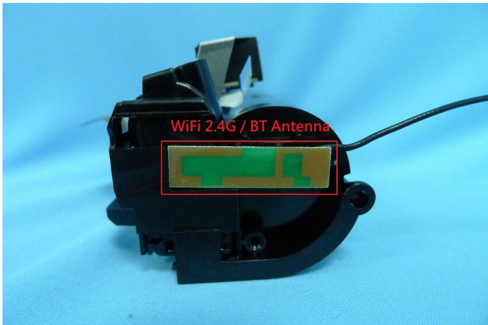
(18) EUT Photo
