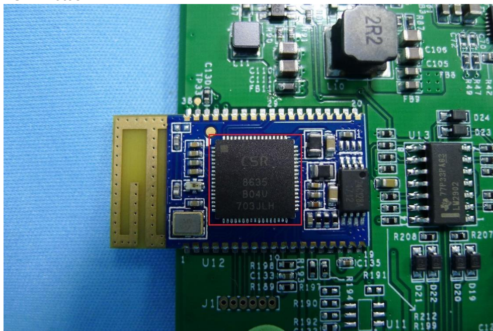
(8) EUT Photos
