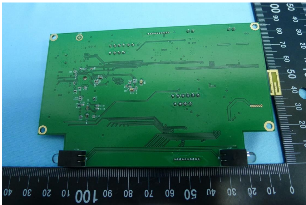
(7) EUT Photos
