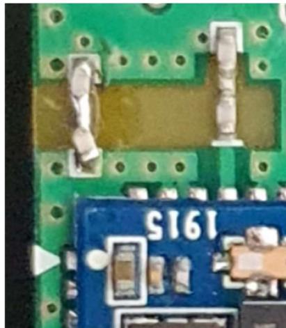
Antenna
