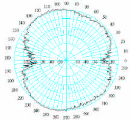
5.15~E-PLANE
