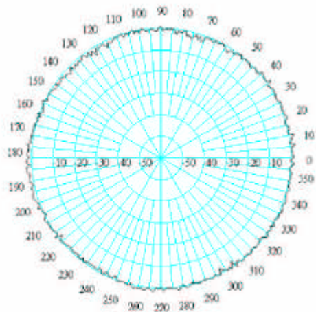
5.15~H-PLANE
