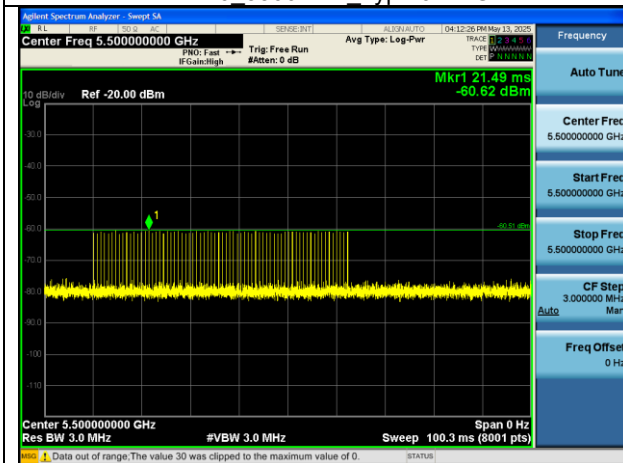
EHT20_5500MHz_Type1-B.PNG
