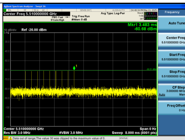
EHT40 5510MHz Type 6.PNG
