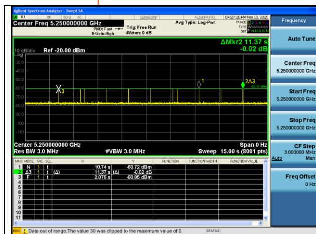
EHT160 5250MHz Type 5.PNG
