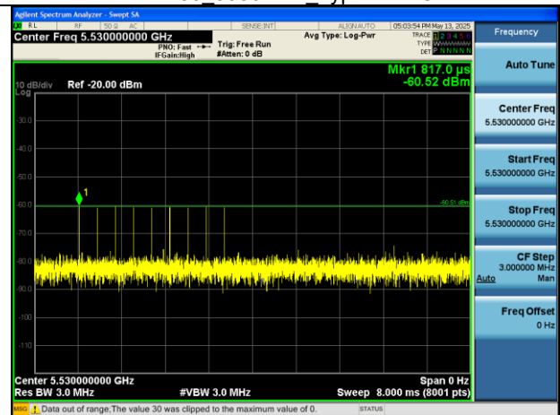
EHT80 5530MHz Type 6.PNG
