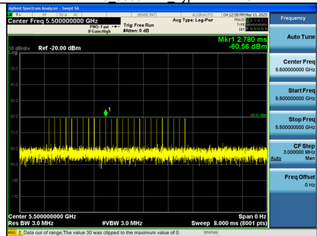
EHT20_5500MHz_Type2.PNG
