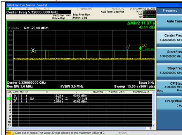
EHT20_5320MHz_Type5.PNG
