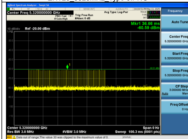
EHT20 5320MHz Type 1-B.PNG
