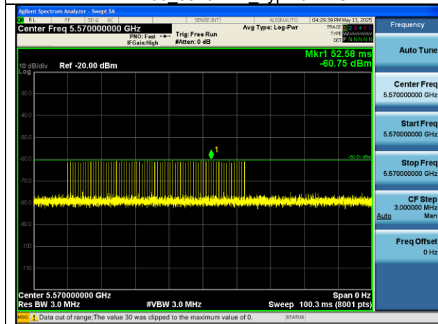
EHT160 5570MHz Type 1-B.PNG
