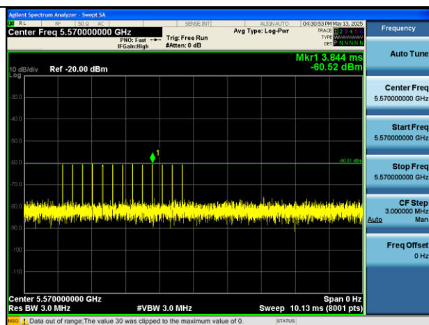
EHT160_5570MHz_Type 4.PNG
