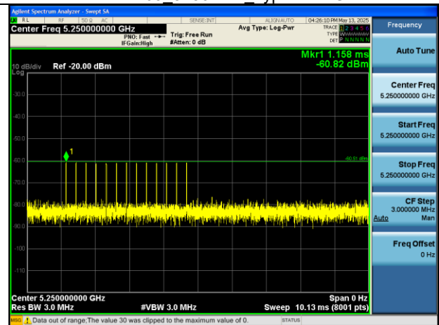
EHT160 5250MHz Type 4.PNG
