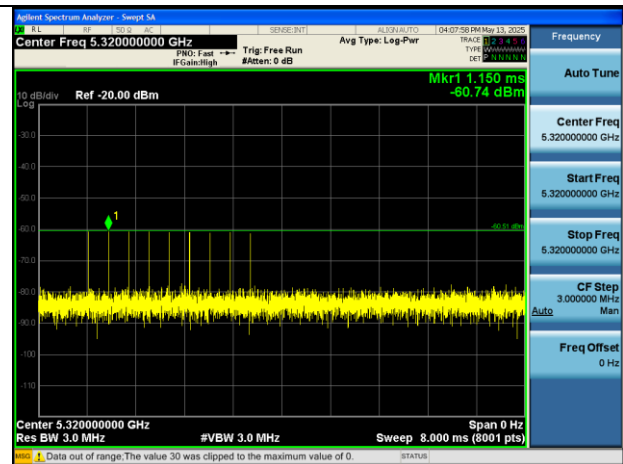
EHT20_5320MHz_Type6.PNG
