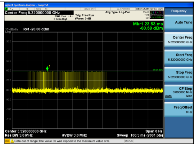
EHT20 5320MHz Type 1-A.PNG
