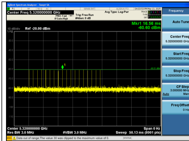
EHT20 5320MHz Type 0.PNG
