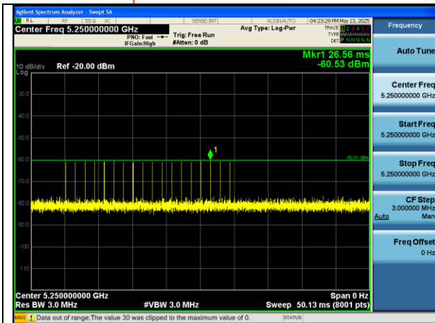
EHT160 5250MHz Type 0.PNG
