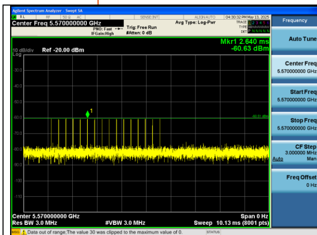
EHT160_5570MHz_Type 3.PNG
