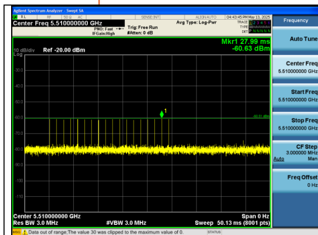
EHT40 5510MHz Type 0.PNG
