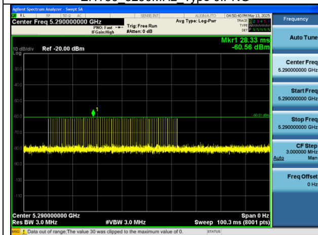
EHT80 5290MHz Type 1-B.PNG
