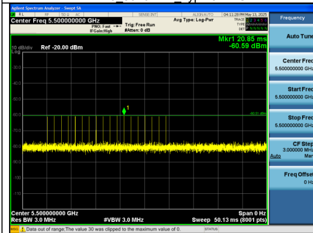
EHT20_5500MHz_Type0.PNG
