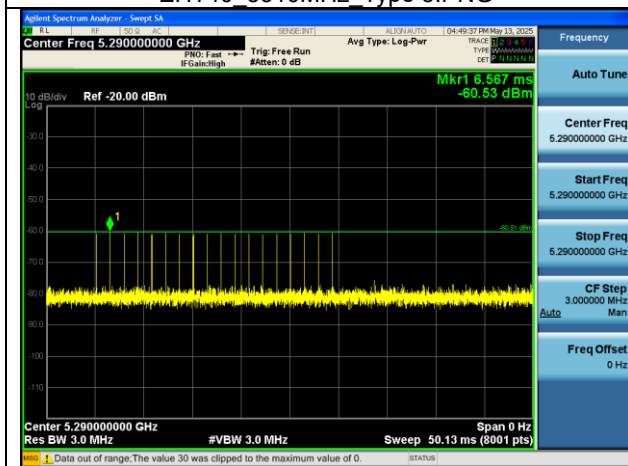
EHT80 5290MHz Type 0.PNG
