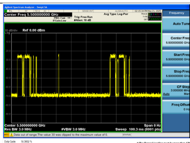
EHT20_5500MHz_Duty Cycle
