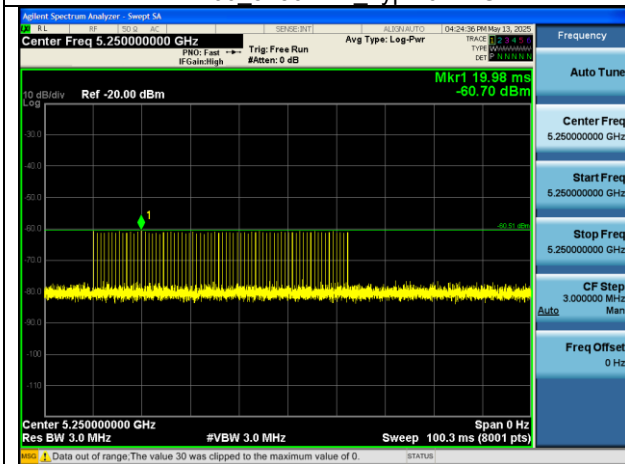
EHT160 5250MHz Type 1-B.PNG
