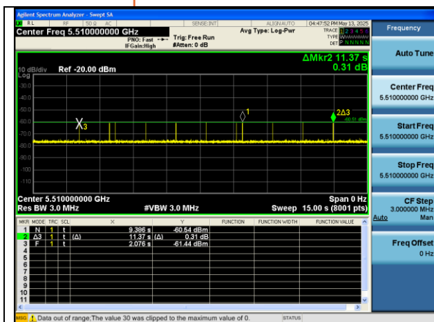
EHT40 5510MHz Type 5.PNG
