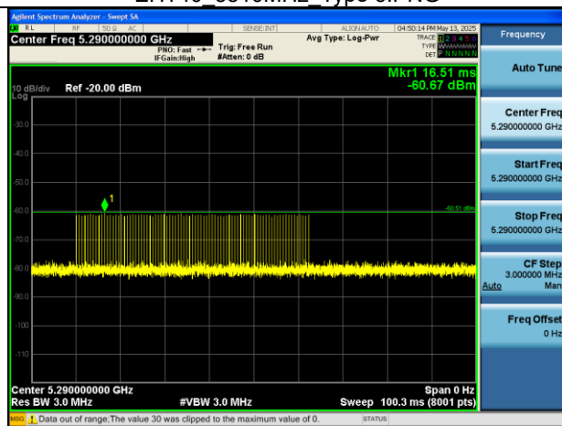
EHT80 5290MHz Type 1-A.PNG
