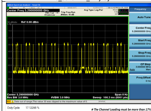
EHT80_5290MHz_Duty Cycle
