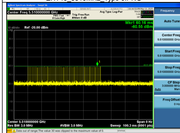
EHT40 5510MHz Type 1-B.PNG
