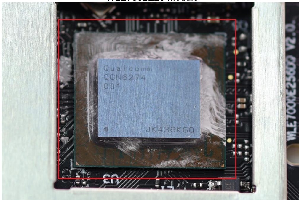
WLE7002E26 Module
