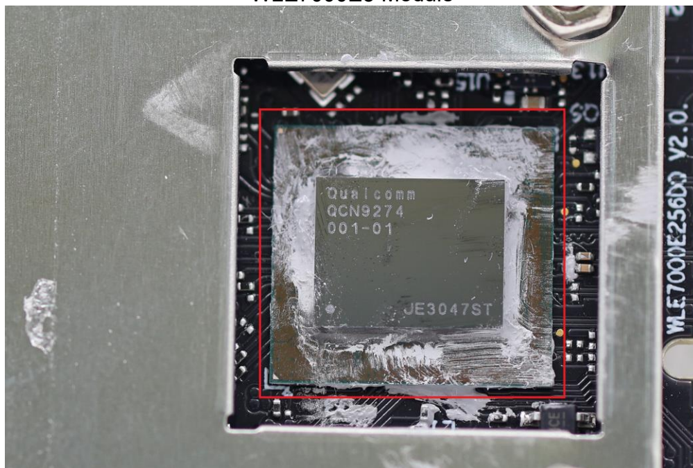
WLE7000E5 Module
