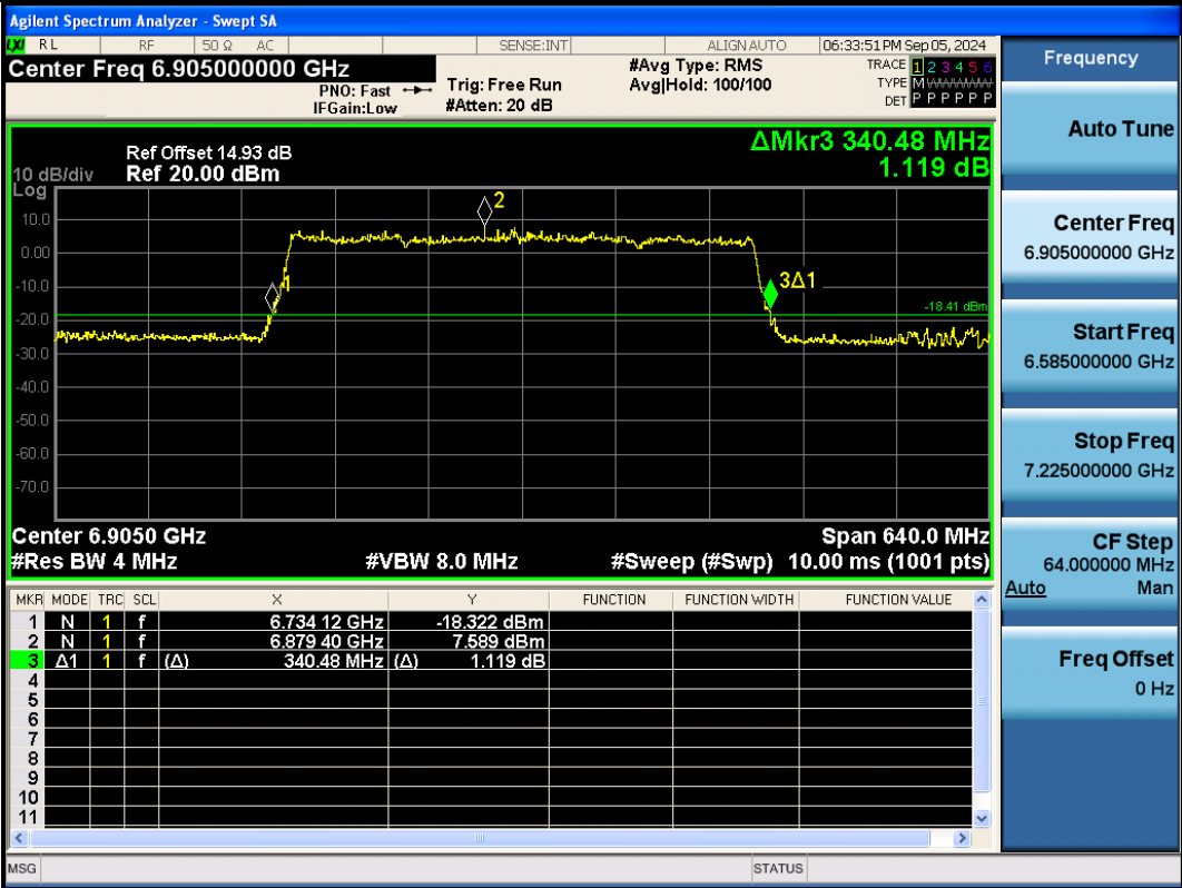
11BE320SISO-Ant1-6905
