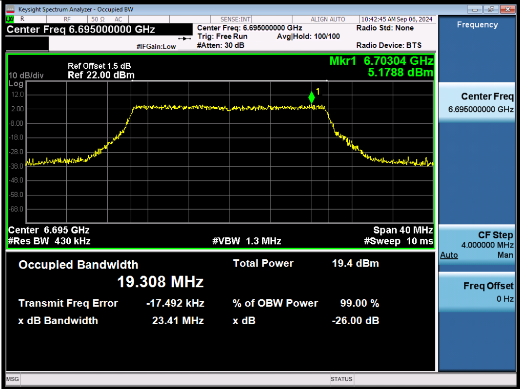
11BE20SISO-Ant1-6695-PASS
