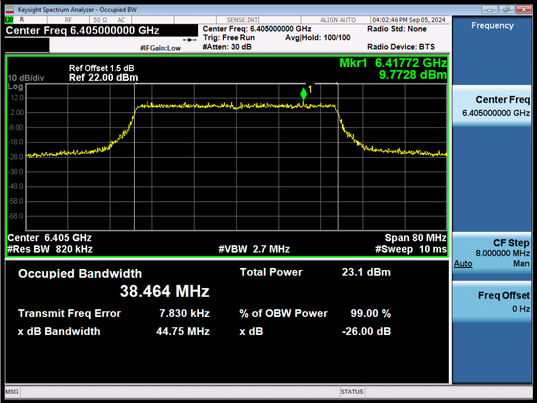
11AX40SISO-Ant1-6405-PASS
