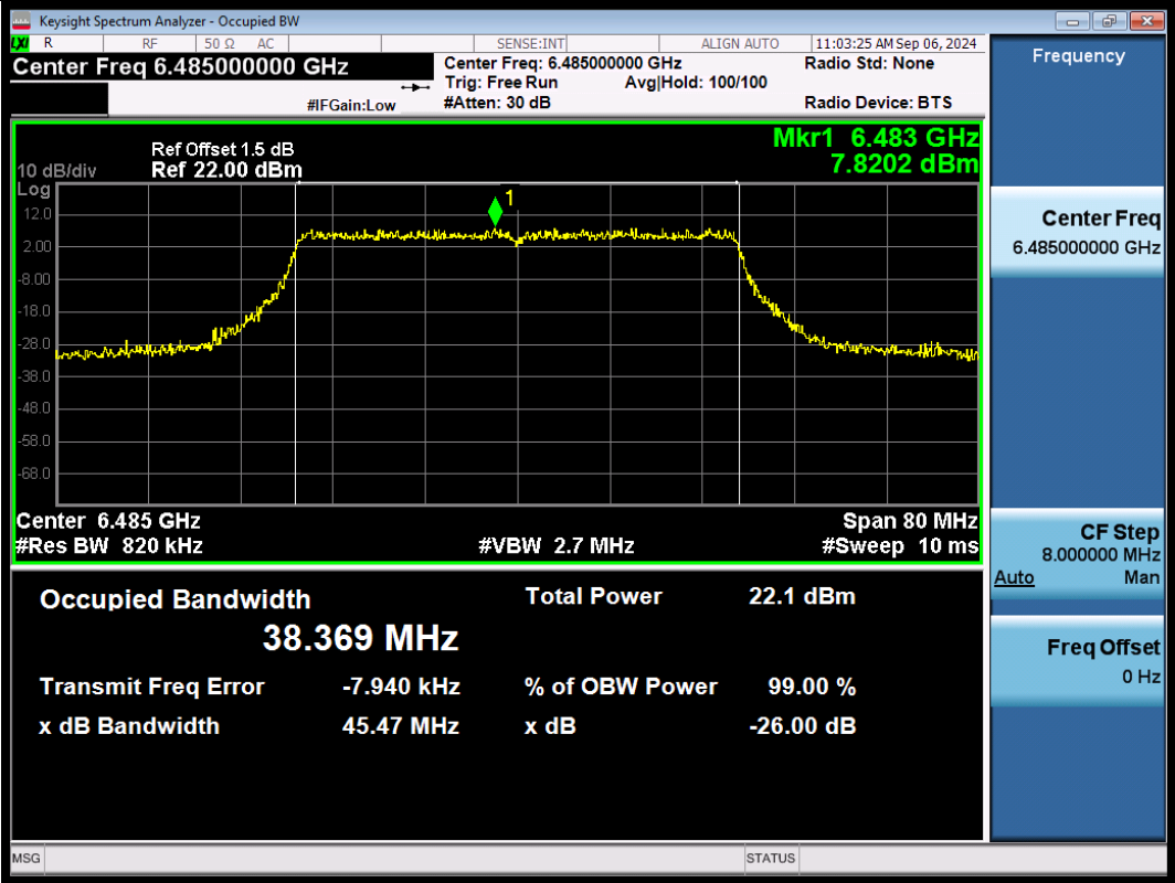
11BE40SISO-Ant1-6485-PASS
