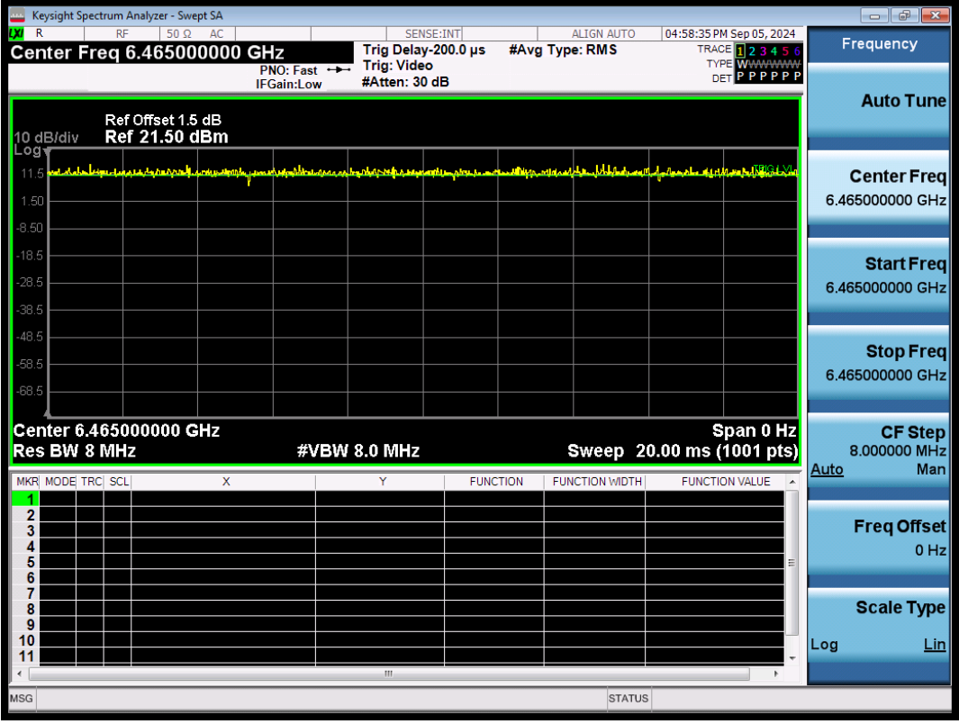
NTNV-11AX80SISO-Ant1-6465
