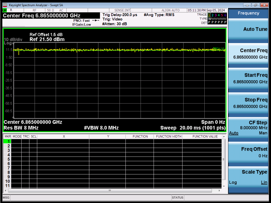
NTNV-11AX80SISO-Ant1-6865
