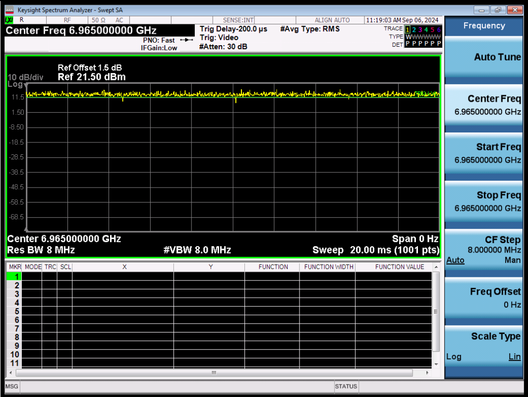
NTNV-11BE40SISO-Ant1-6965
