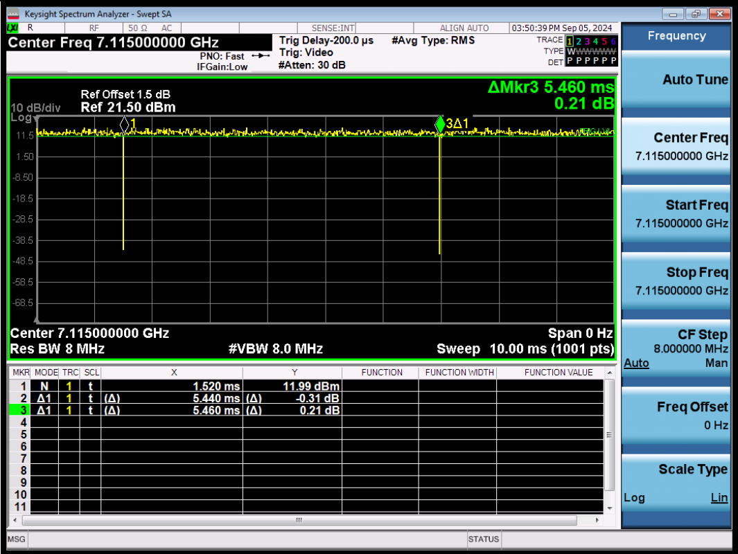
NTNV-11AX20SISO-Ant1-7115
