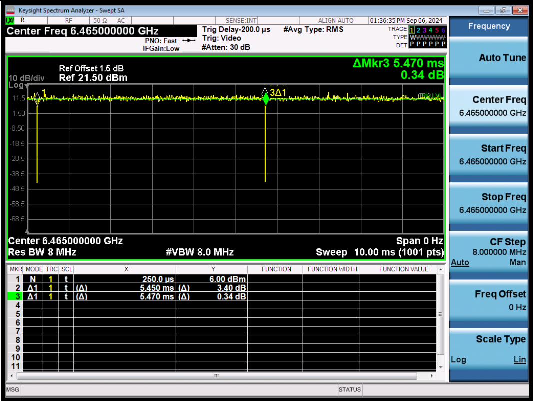
NTNV-11BE80SISO-Ant1-6465
