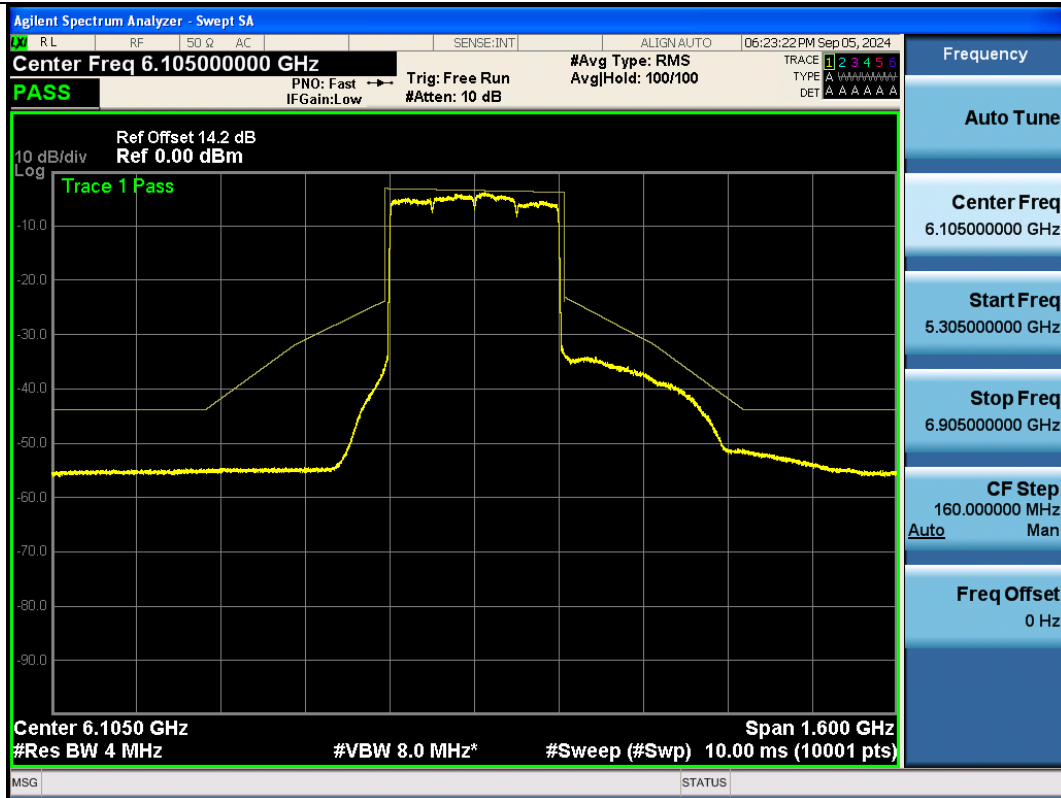
NTNV-11BE320SISO-Ant1-6105-PASS
