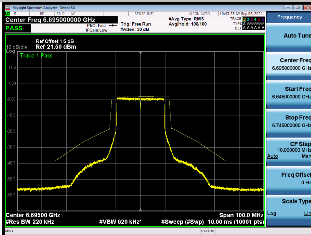
NTNV-11BE20SISO-Ant1-6695-PASS
