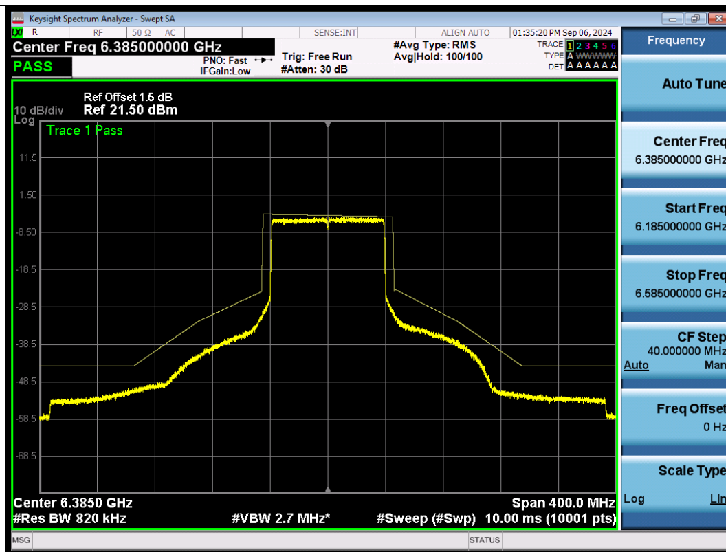
NTNV-11BE80SISO-Ant1-6385-PASS
