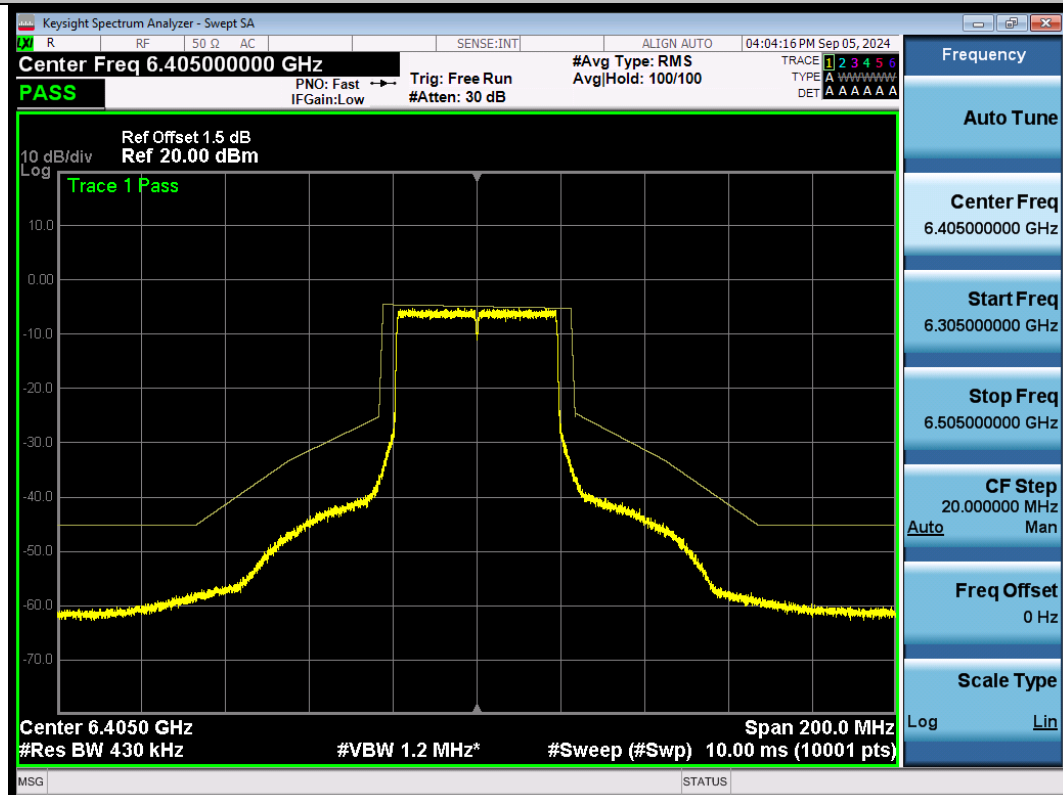
NTNV-11AX40SISO-Ant1-6405-PASS
