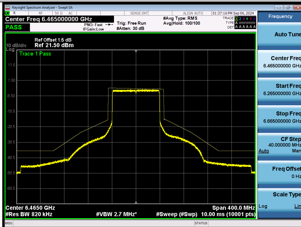
NTNV-11BE80SISO-Ant1-6465-PASS
