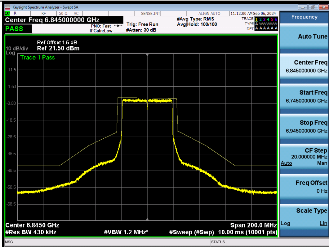
NTNV-11BE40SISO-Ant1-6845-PASS
