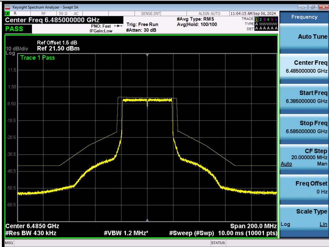
NTNV-11BE40SISO-Ant1-6485-PASS
