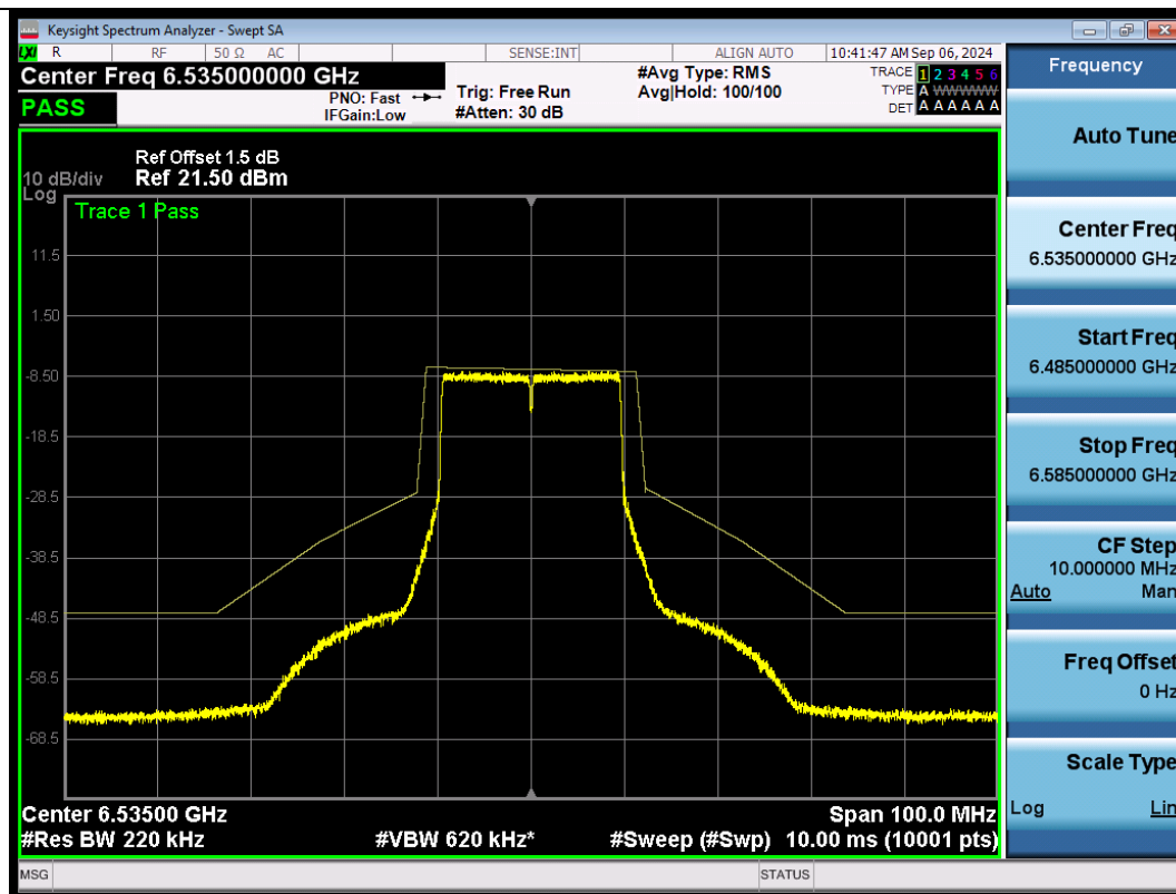
NTNV-11BE20SISO-Ant1-6535-PASS
