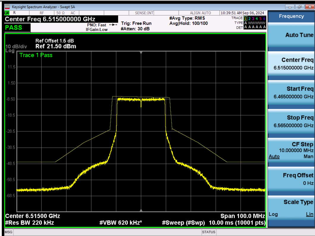
NTNV-11BE20SISO-Ant1-6515-PASS
