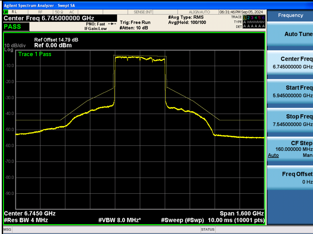
NTNV-11BE320SISO-Ant1-6745-PASS
