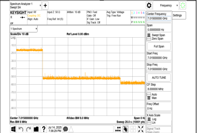
802.11be_20MHz_7015MHz_Interference_7015MHz_-73.11dBm_OFF
