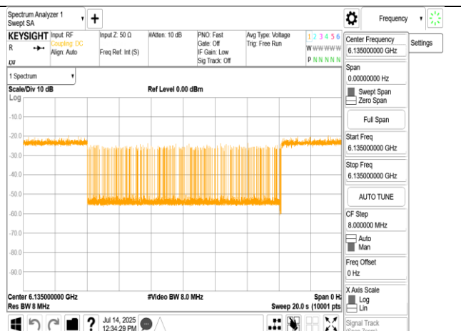
802.11be_20MHz_6135MHz_Interference_6135MHz_ - 75.14dBm Minimal
