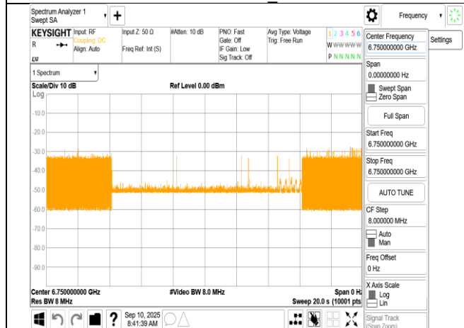
802.11be_320MHz_6905MHz_Interference_6750MHz_- 70.24dBm_Minimal
