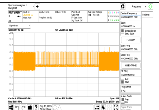
802.11be_320MHz_6265MHz_Interference_6420MHz_- 73.32dBm_Minimal
