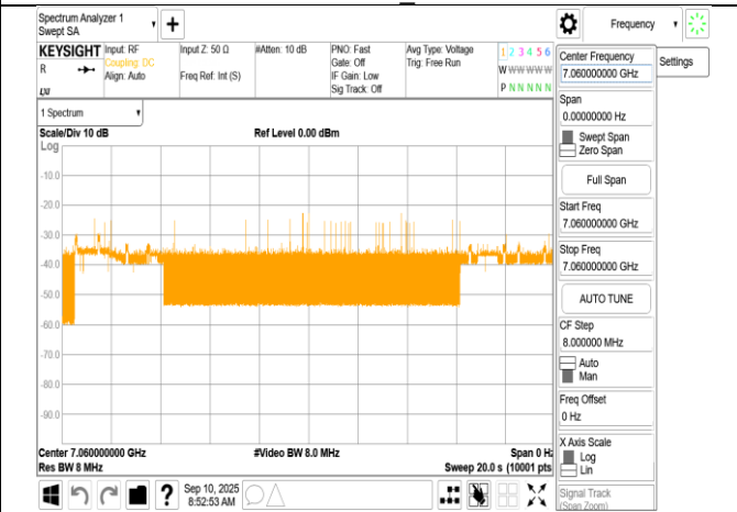
802.11be_320MHz_6905MHz_Interference_7060MHz_- 73.23dBm_ON
