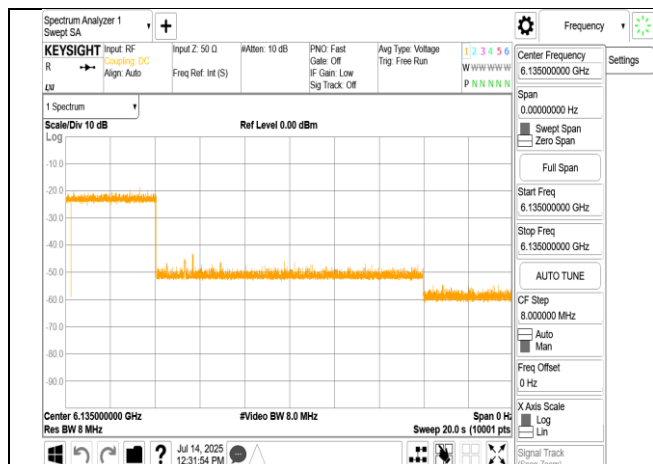
802.11be_20MHz_6135MHz_Interference_6135MHz_ - 71.14dBm OFF
