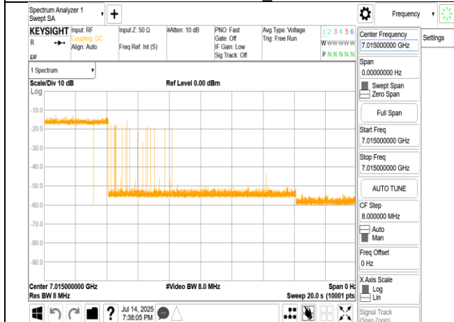
802.11be_20MHz_7015MHz_Interference_7015MHz_-76.11dBm_Minimal
