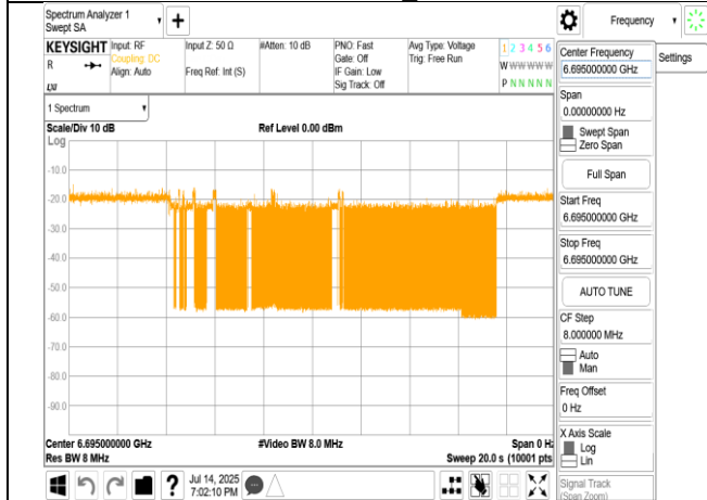
802.11be_20MHz_6695MHz_Interference_6695MHz_-79.24dBm_ON
