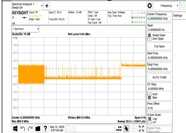
802.11be_320MHz_6265MHz_Interference_6265MHz_- 73.17dBm_Minimal
