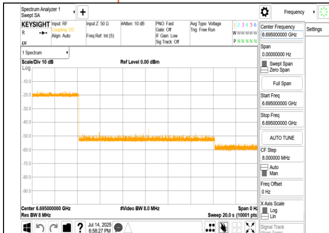
802.11be_20MHz_6695MHz_Interference_6695MHz_-73.24dBm_OFF
