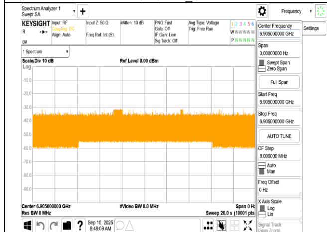
802.11be_320MHz_6905MHz_Interference_6905MHz_- 76.15dBm_ON
