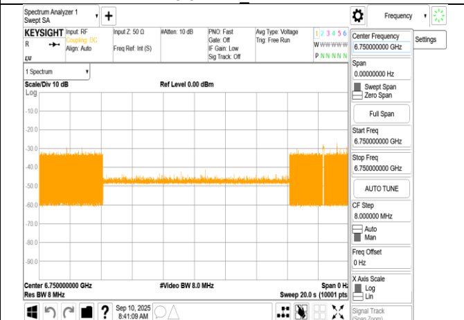
802.11be_320MHz_6905MHz_Interference_6750MHz_- 67.24dBm_OFF
