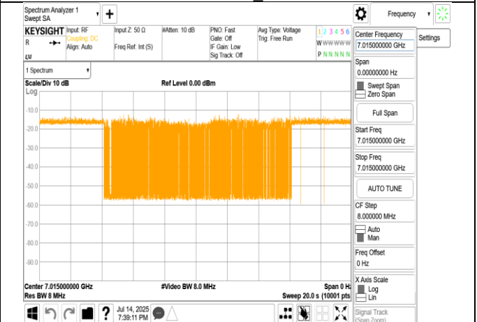
802.11be_20MHz_7015MHz_Interference_7015MHz_-79.11dBm_ON
