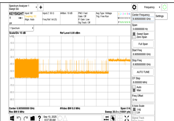
802.11be_320MHz_6905MHz_Interference_6905MHz_- 73.15dBm_Minimal
