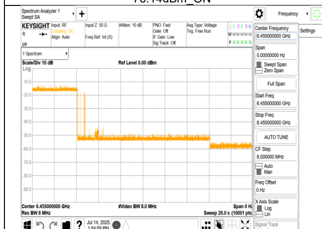
802.11be_20MHz_6455MHz_Interference_6455MHz_ - 73.14dBm Minimal
