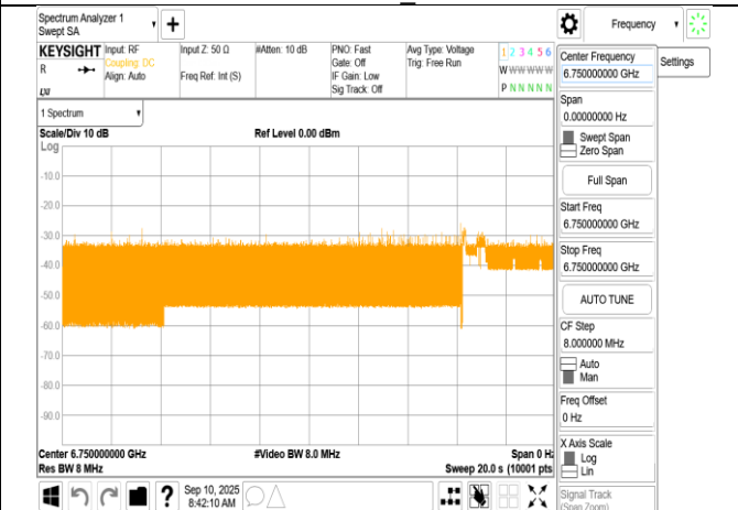
802.11be_320MHz_6905MHz_Interference_6750MHz_- 73.24dBm_ON
