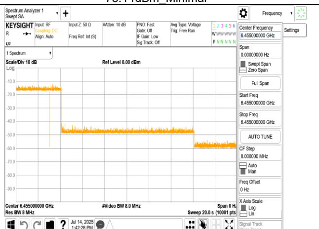
802.11be_20MHz_6455MHz_Interference_6455MHz_ - 67.14dBm OFF
