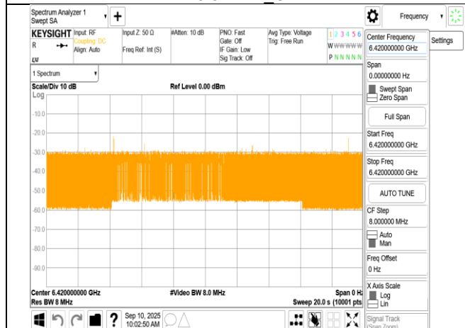
802.11be_320MHz_6265MHz_Interference_6420MHz_- 76.32dBm_ON
