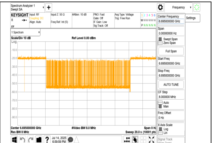
802.11be_20MHz_6695MHz_Interference_6695MHz_-76.24dBm_Minimal
