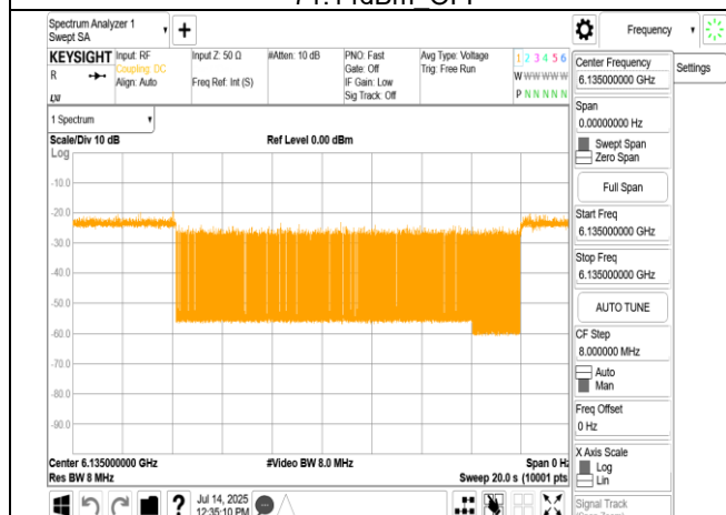
802.11be_20MHz_6135MHz_Interference_6135MHz_ - 76.14dBm ON
