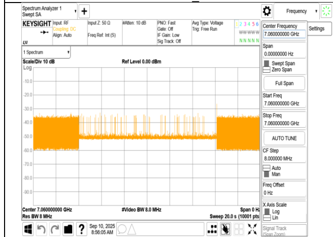
802.11be_320MHz_6905MHz_Interference_7060MHz_- 71.23dBm_Minimal
