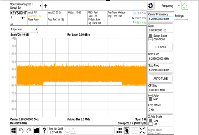
802.11be_320MHz_6265MHz_Interference_6265MHz_- 76.17dBm_ON
