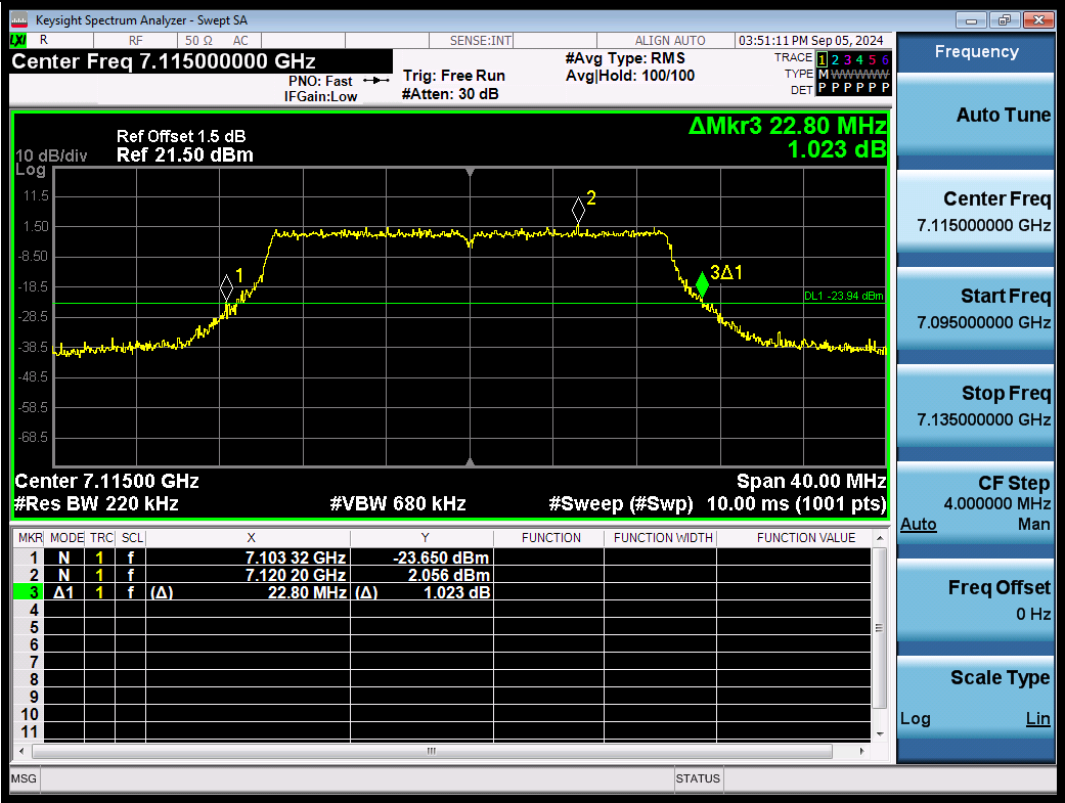
11AX20SISO-Ant1-7115
