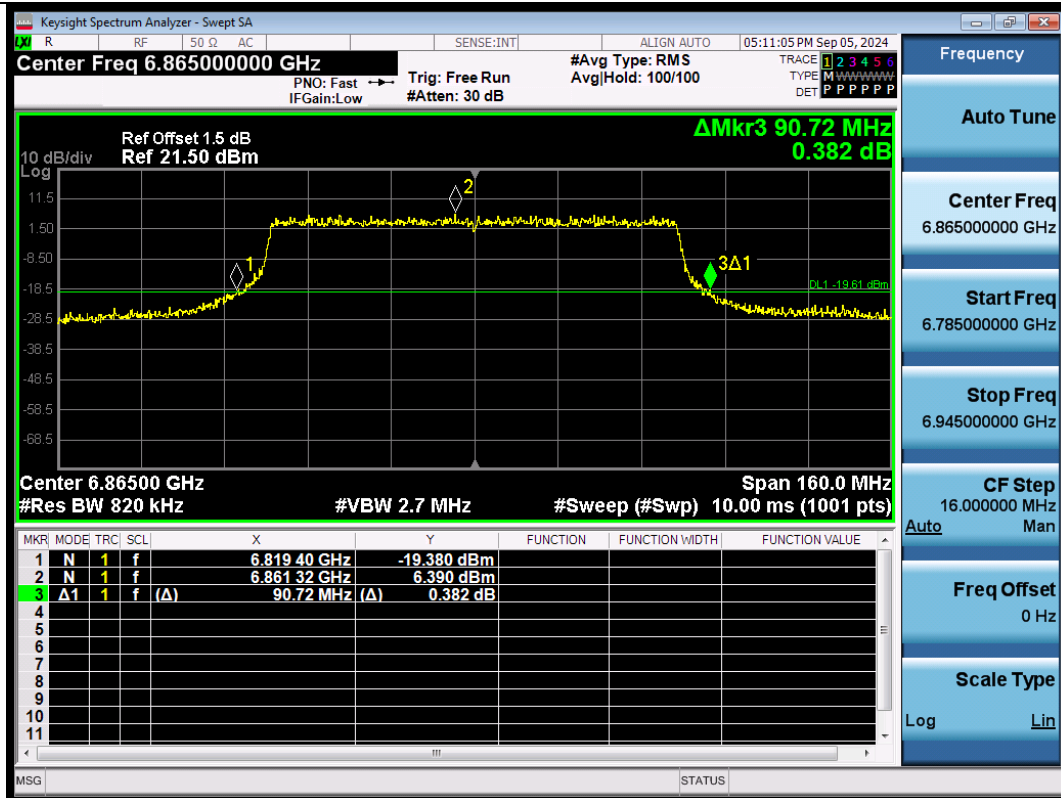
11AX80SISO-Ant1-6865
