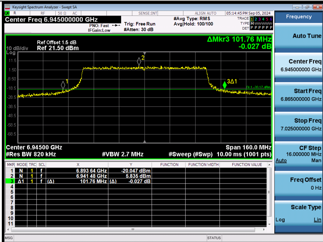
11AX80SISO-Ant1-6945
