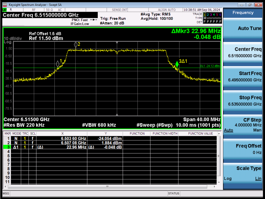
11BE20SISO-Ant1-6515
