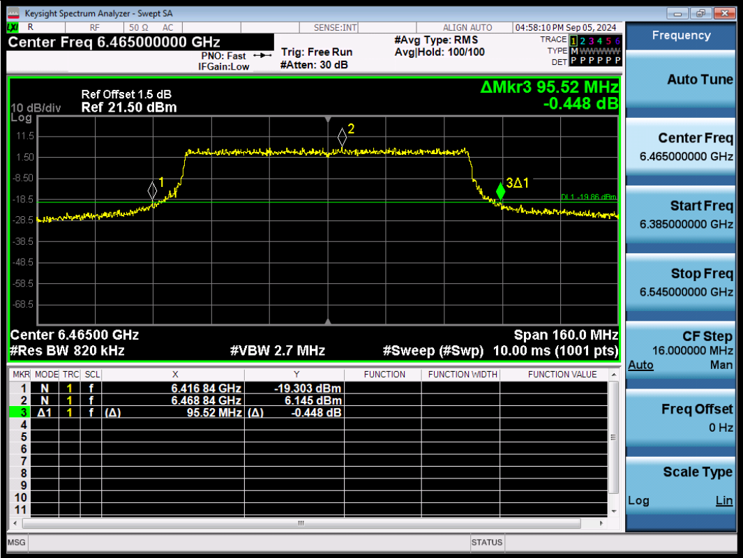
11AX80SISO-Ant1-6465
