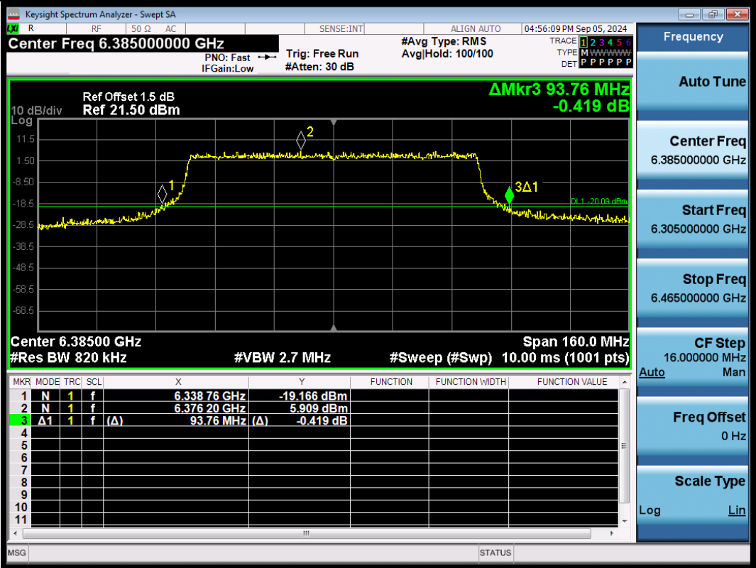
11AX80SISO-Ant1-6385
