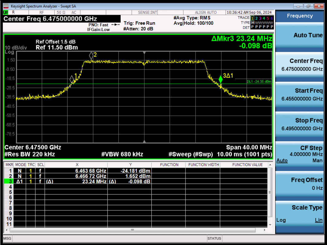
11BE20SISO-Ant1-6475
