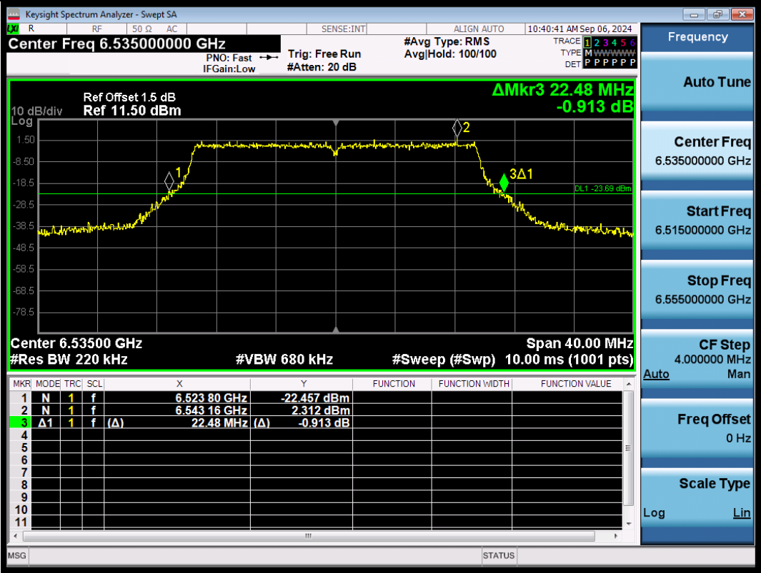
11BE20SISO-Ant1-6535
