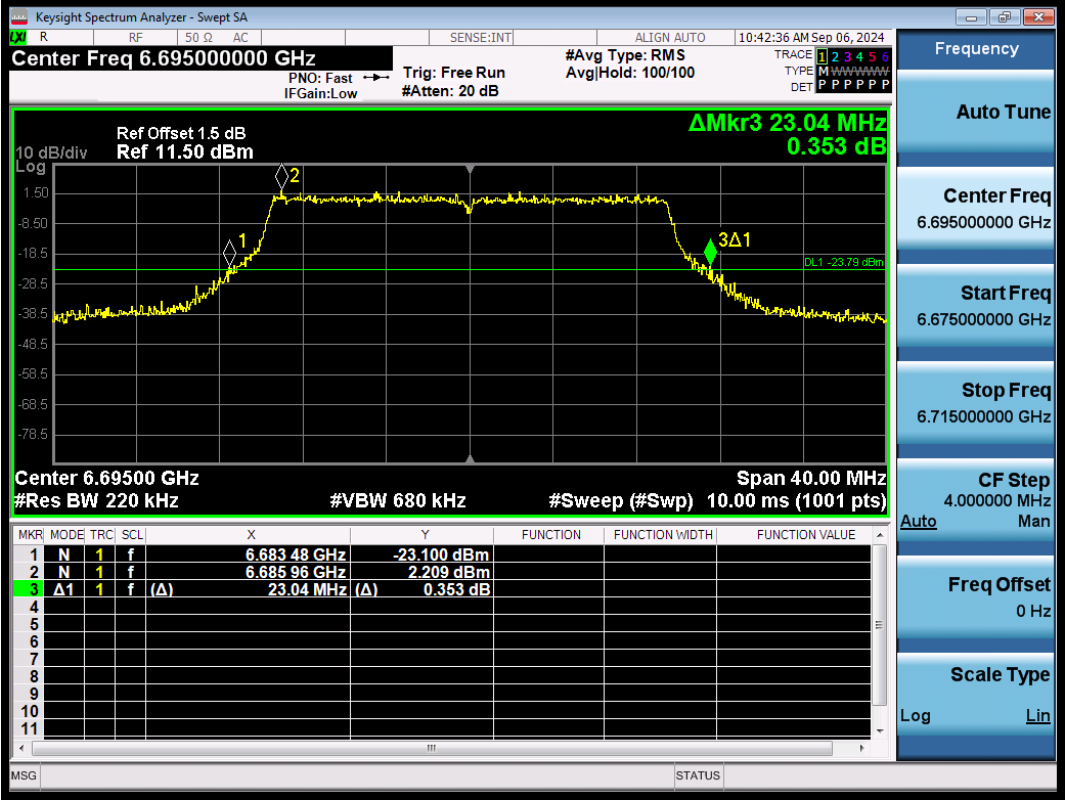
11BE20SISO-Ant1-6695
