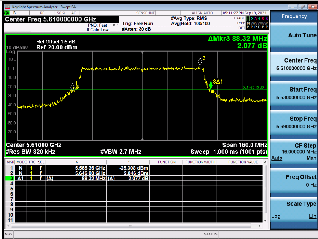
11AX80SISO-Ant1-5610
