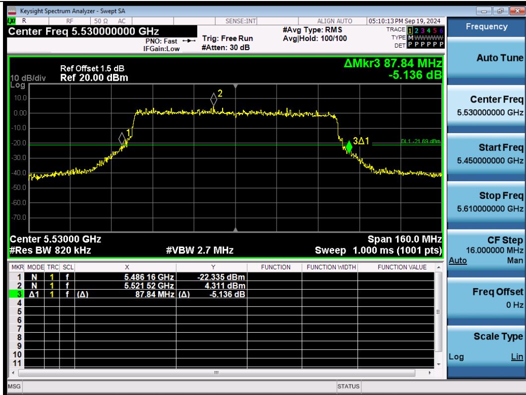
11AX80SISO-Ant1-5530
