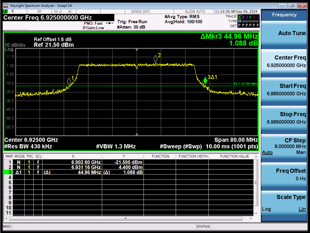
11BE40SISO-Ant1-6925
