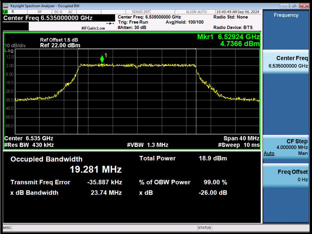
11BE20SISO-Ant1-6535-PASS
