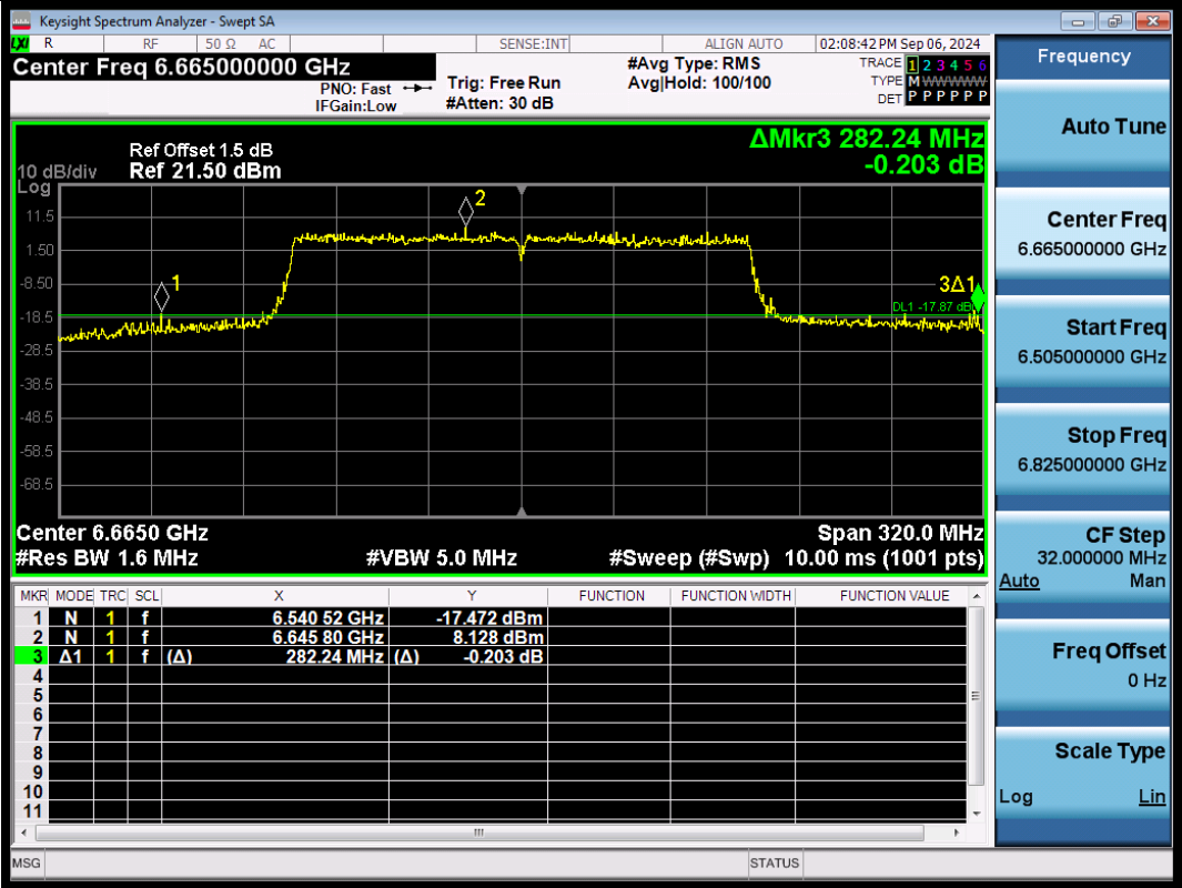
11BE160SISO-Ant1-6665
