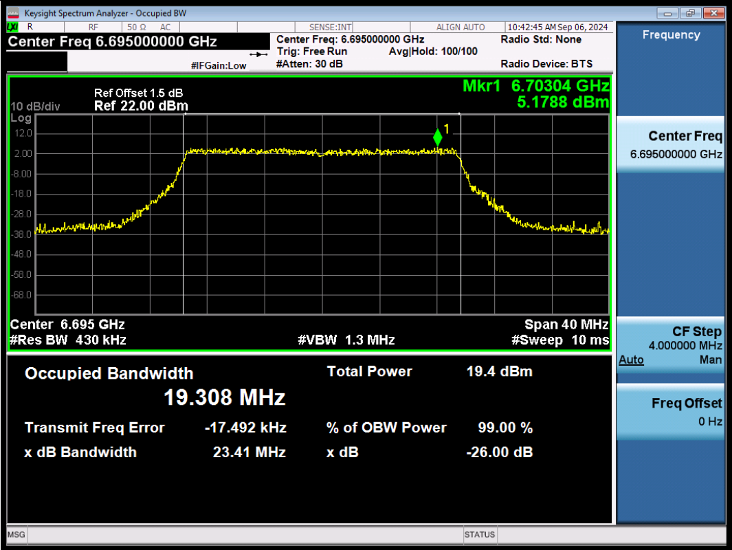
11BE20SISO-Ant1-6695-PASS
