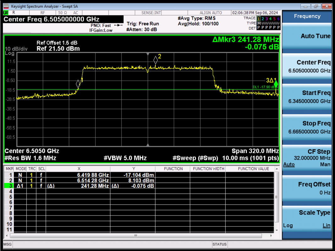
11BE160SISO-Ant1-6505
