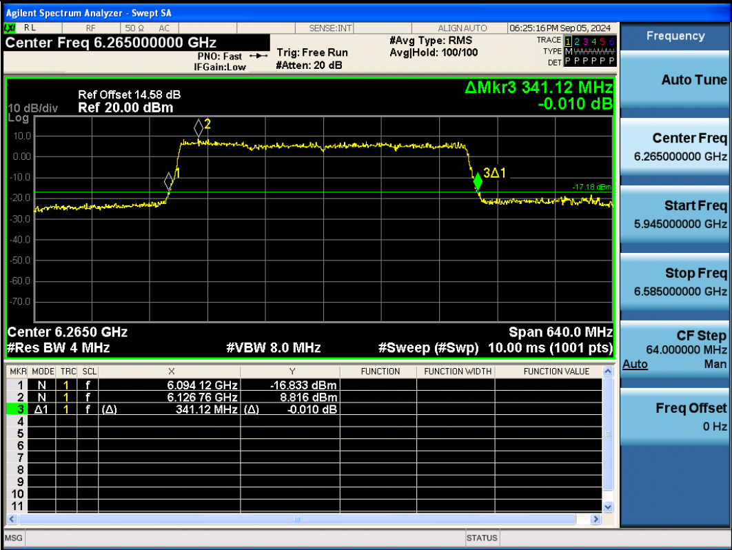
11BE320SISO-Ant1-6265
