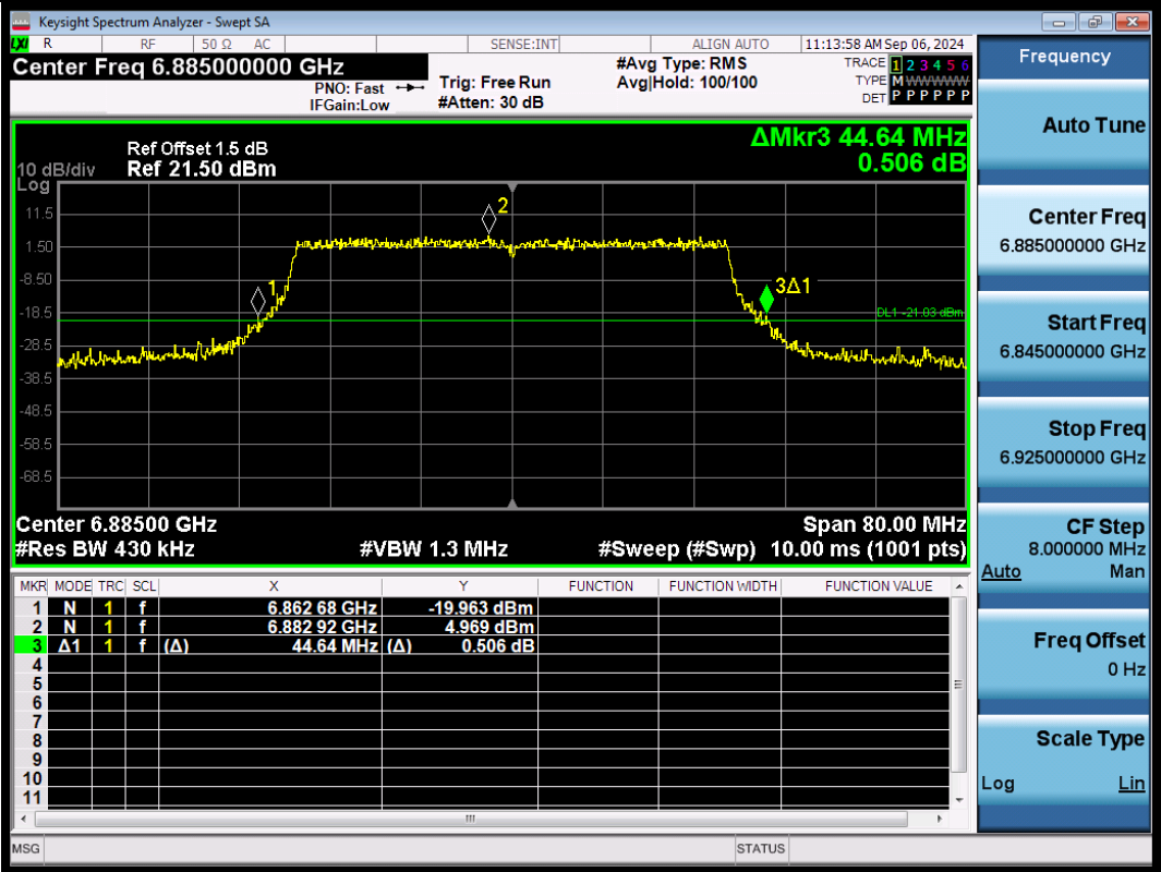
11BE40SISO-Ant1-6885
