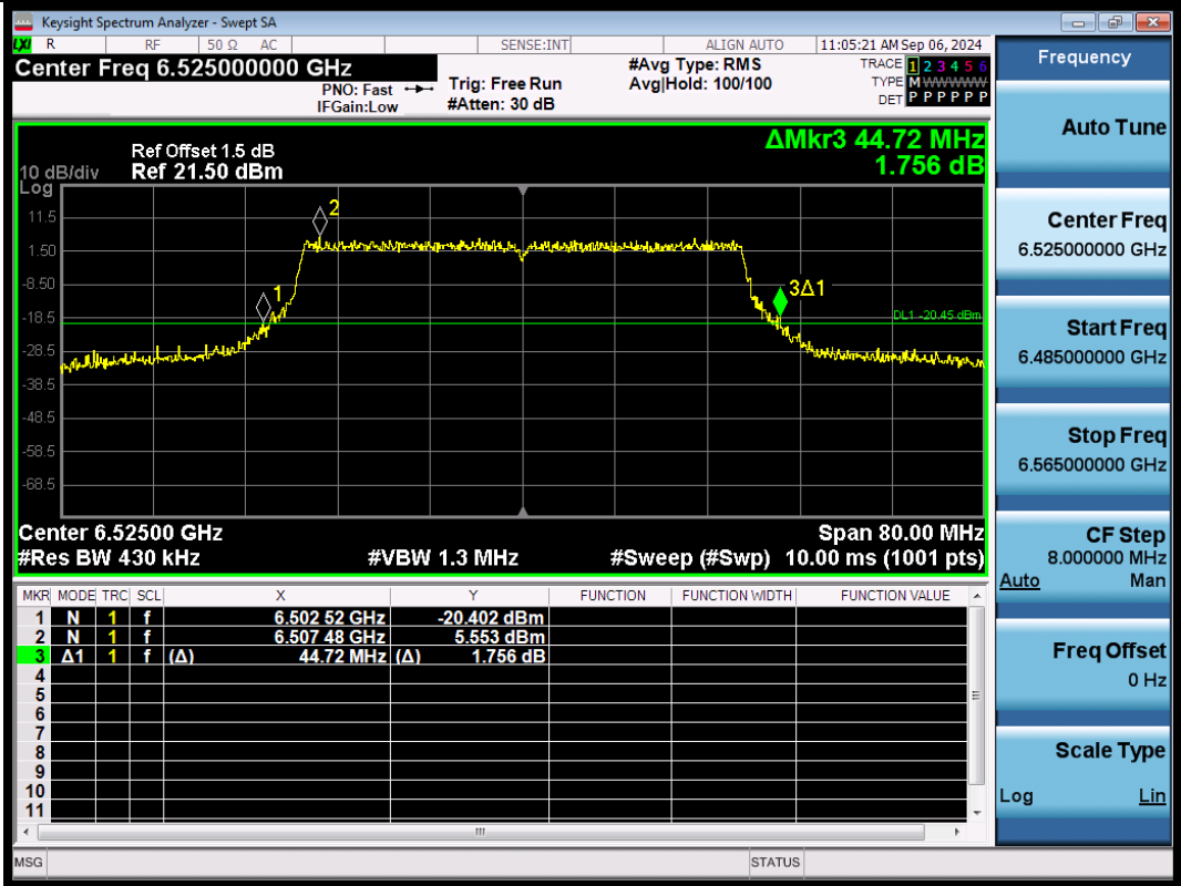
11BE40SISO-Ant1-6525
