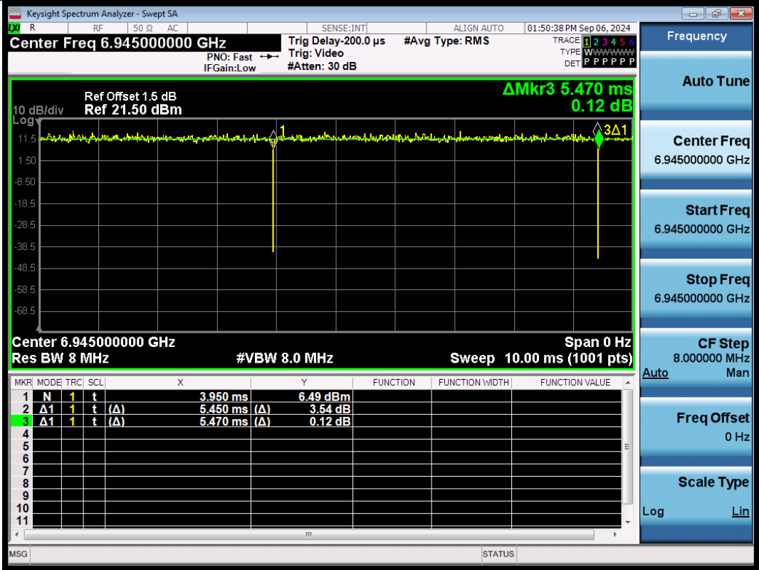
NTNV-11BE80SISO-Ant1-6945
