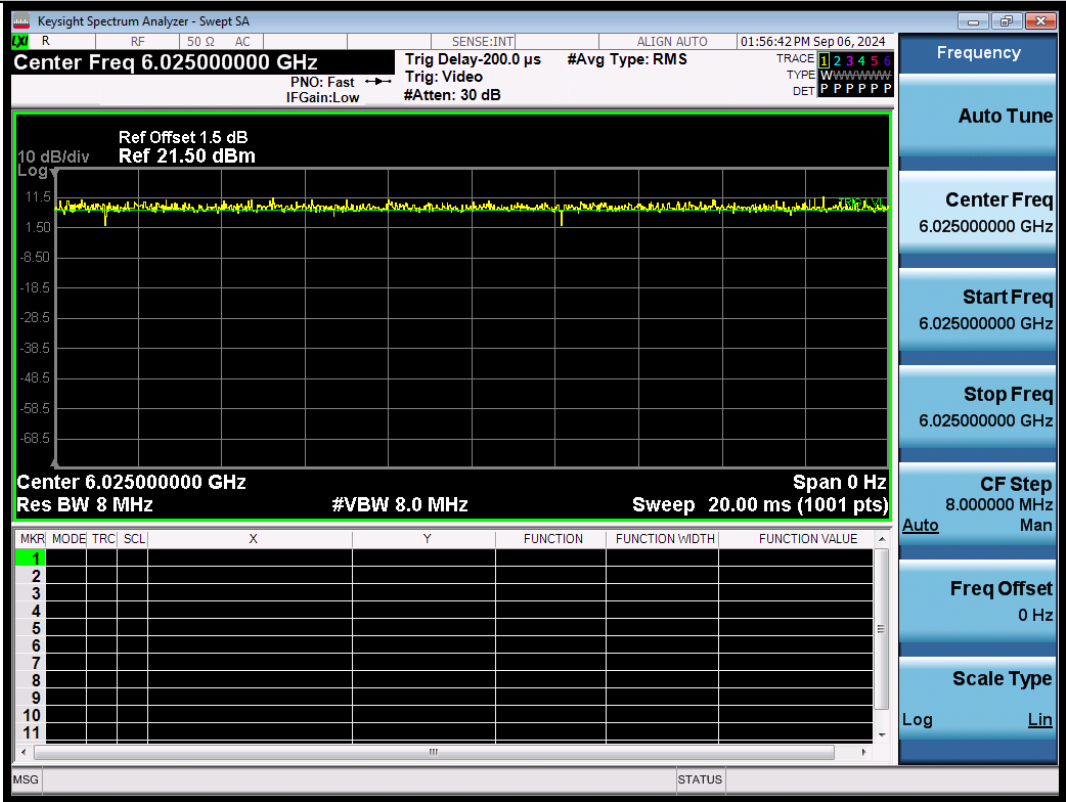
NTNV-11BE160SISO-Ant1-6025
