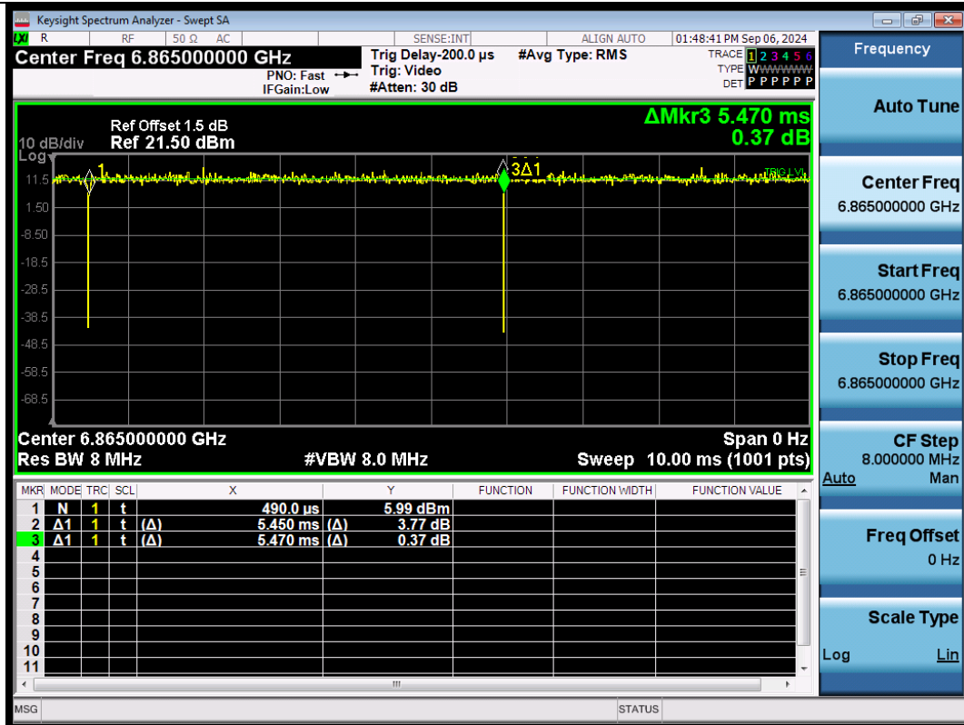
NTNV-11BE80SISO-Ant1-6865
