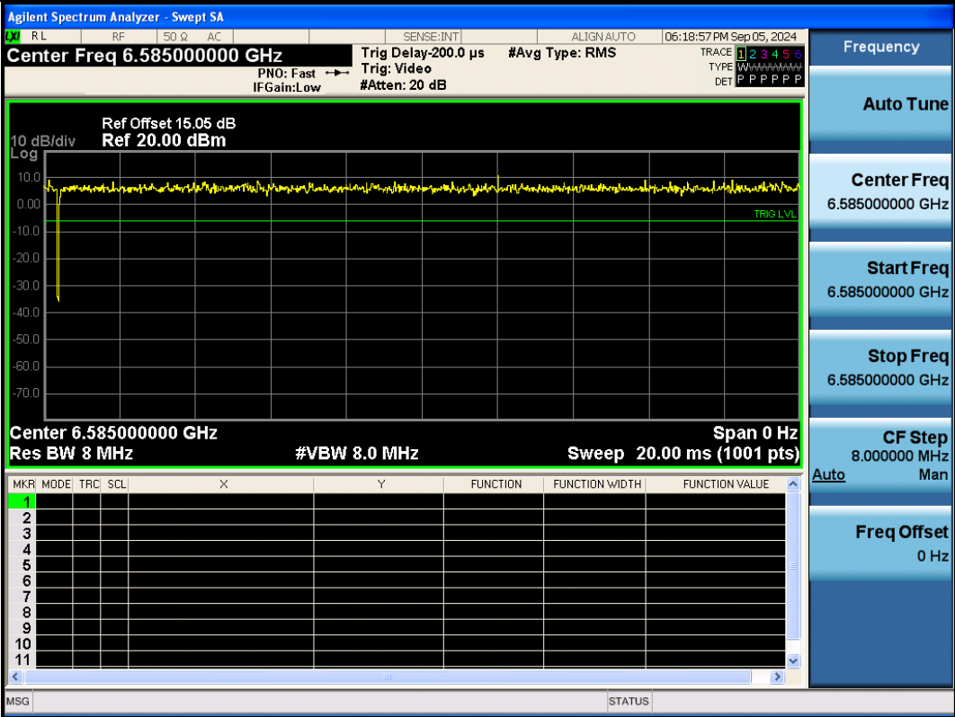
NTNV-11BE320SISO-Ant1-6585
