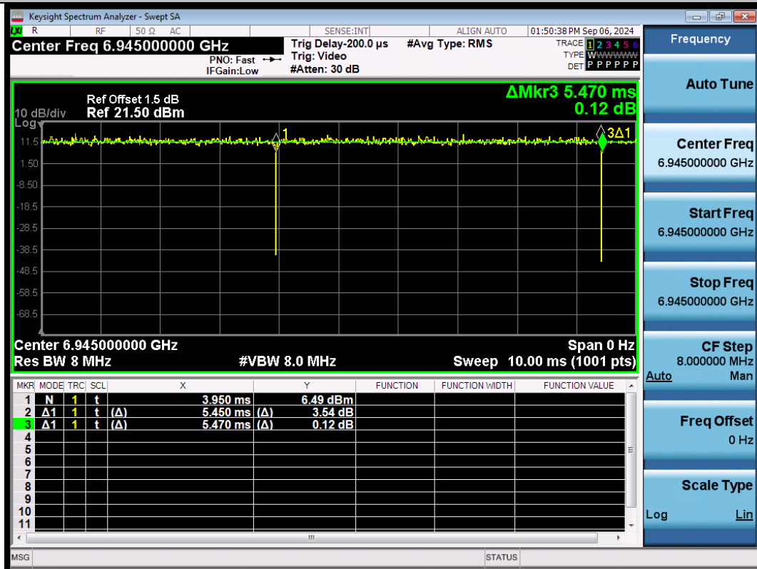
NTNV-11BE80SISO-Ant1-6945
