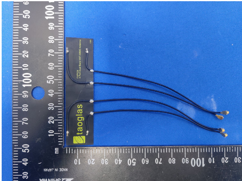
(8) EUT Photo (Antenna 2#)
