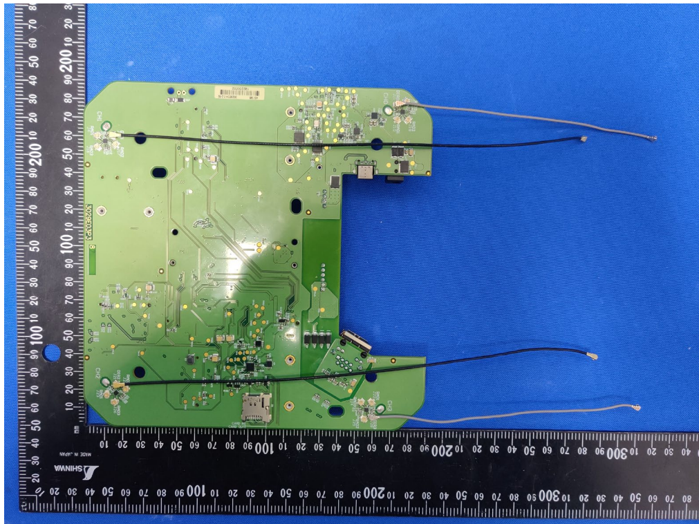
(9) EUT Photo (Antenna 2#)
