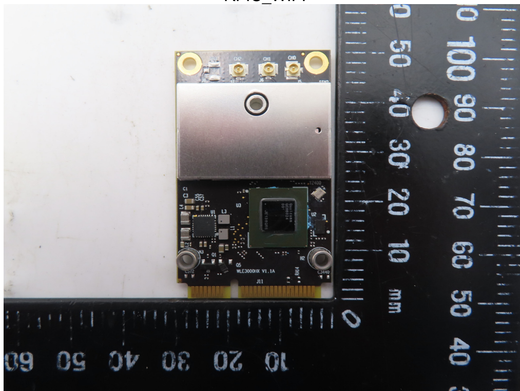
RFIC_WIFI
