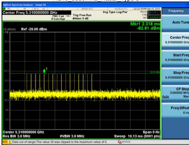
HE40 5310MHz Radar Type 4
