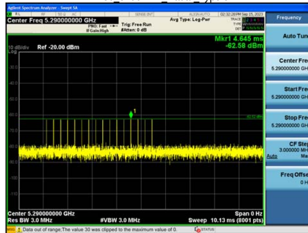
HE80 5290MHz Radar Type 4
