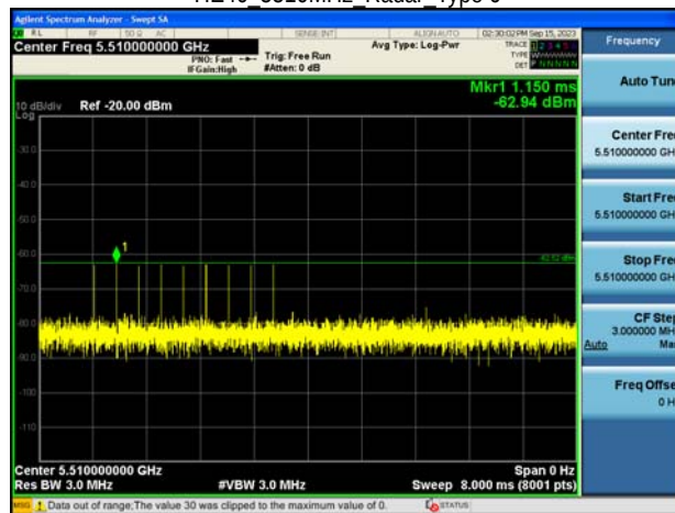
HE40 5510MHz Radar Type 6
