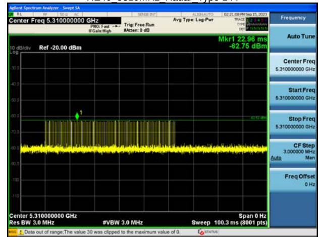
HE40 5310MHz Radar Type 1-B
