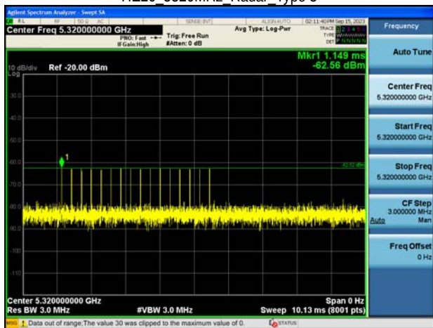
HE20 5320MHz Radar Type 3
