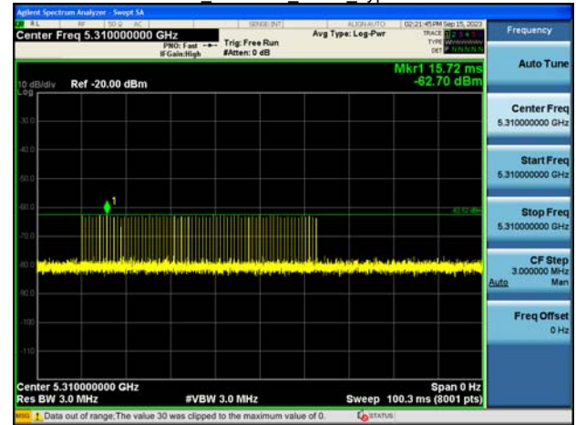
HE40 5310MHz Radar Type 2
