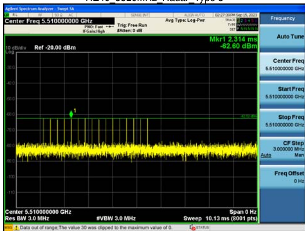
HE40 5510MHz Radar Type 3
