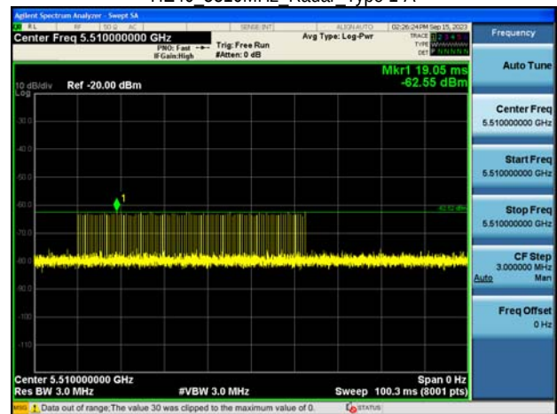
HE40 5510MHz Radar Type 1-A
