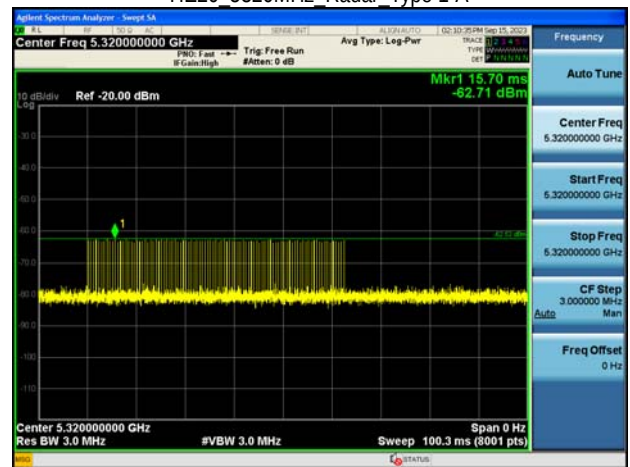
HE20 5320MHz Radar Type 1-A
