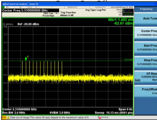
HE40 5310MHz Radar Type 5
