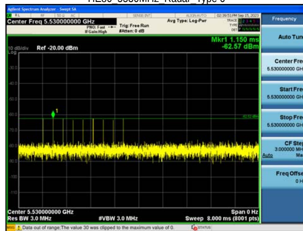
HE80 5530MHz Radar Type 6
