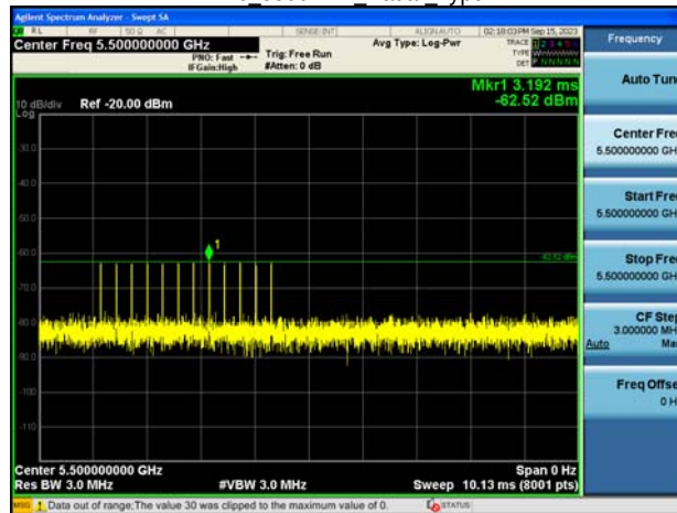
HE20 5500MHz Radar Type 4
