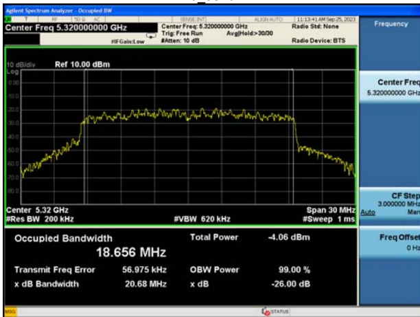
HE20 5320MHz
