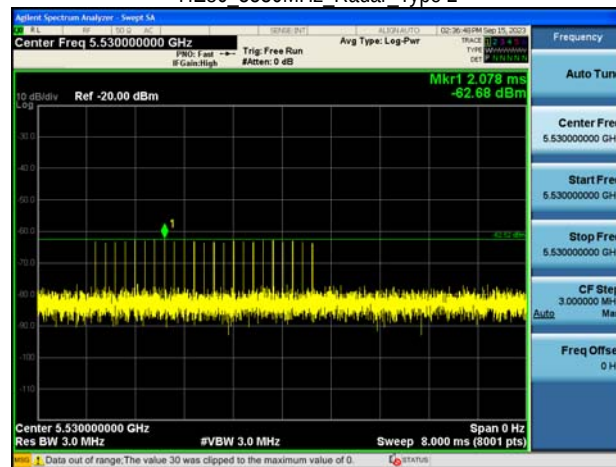
HE80 5530MHz Radar Type 2
