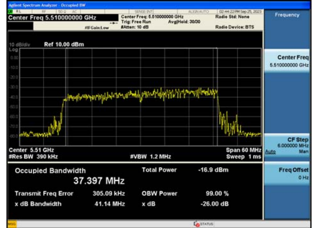
HE40 5510MHz
