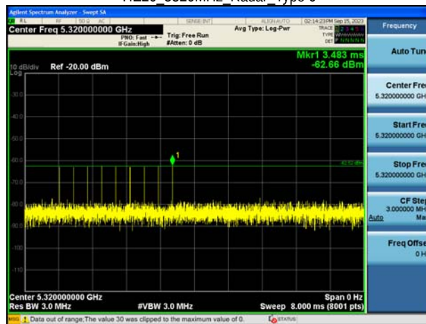
HE20 5320MHz Radar Type 6
