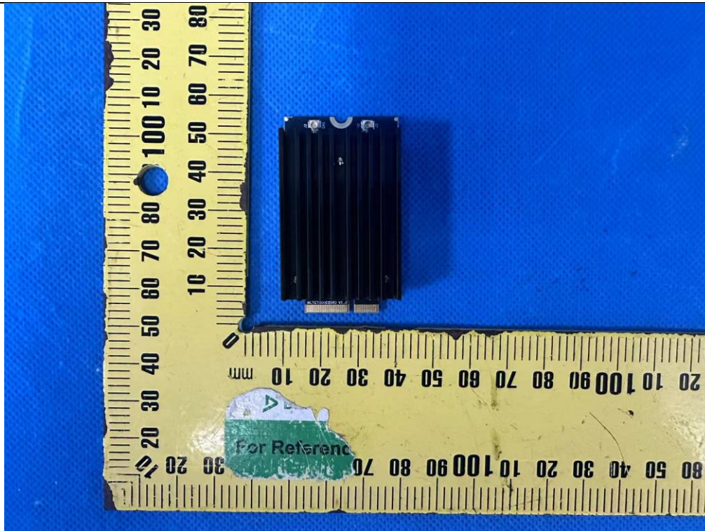
EUT Photo(6) - WLTE7002E25
