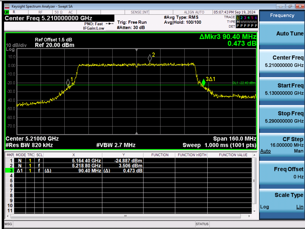
11AX80SISO-Ant1-5210
