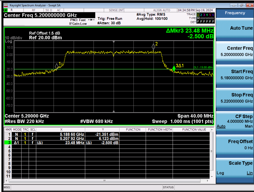
11AX20SISO-Ant1-5200
