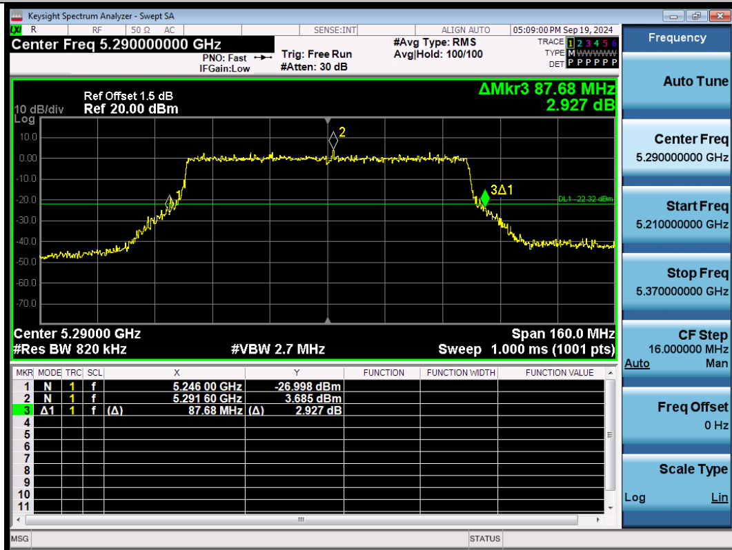
11AX80SISO-Ant1-5290
