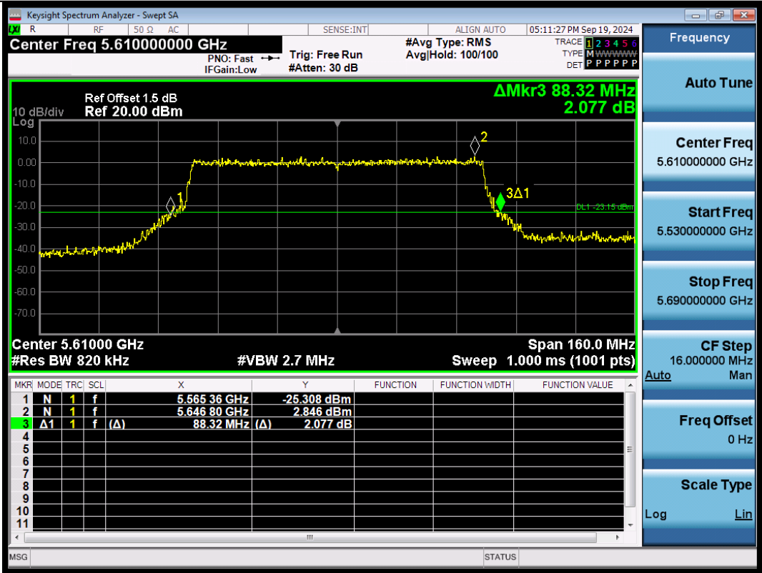
11AX80SISO-Ant1-5610
