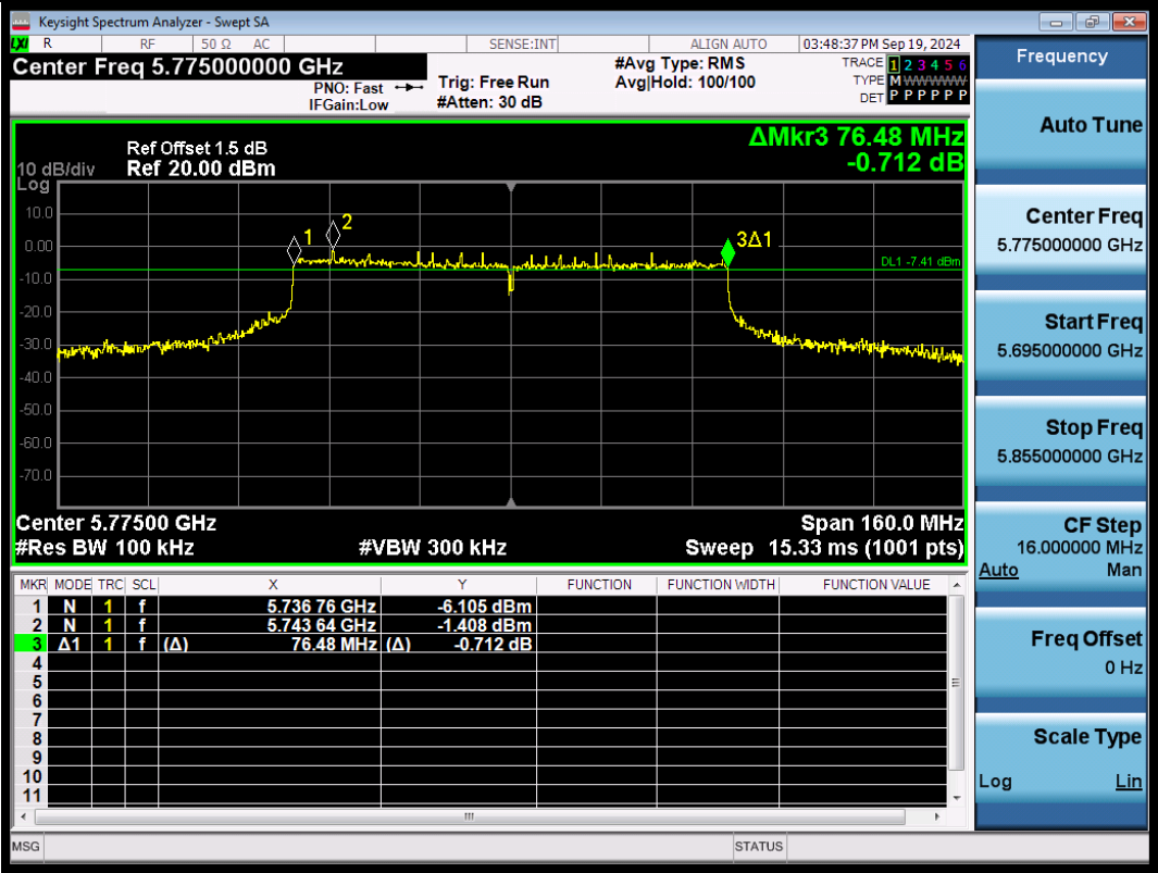
11AC80SISO-Ant1-5775-PASS
