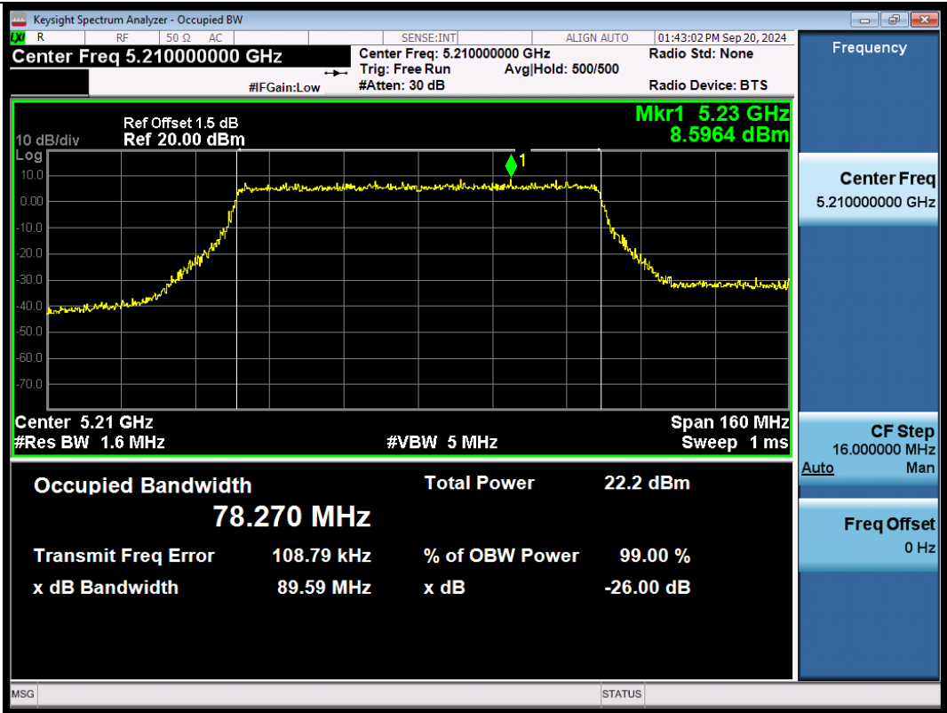
11BE80SISO-Ant1-5210
