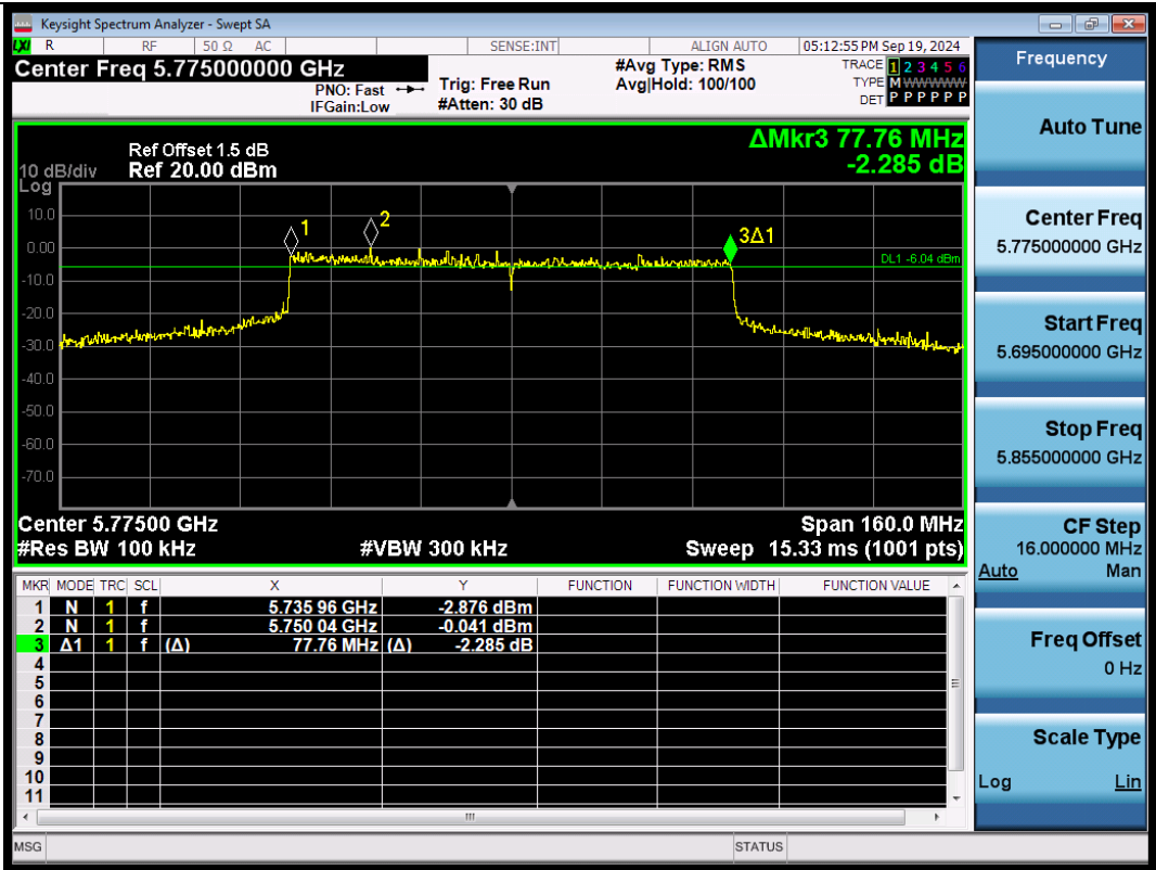
11AX80SISO-Ant1-5775-PASS
