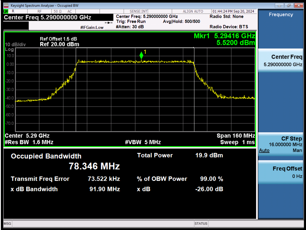
11BE80SISO-Ant1-5290
