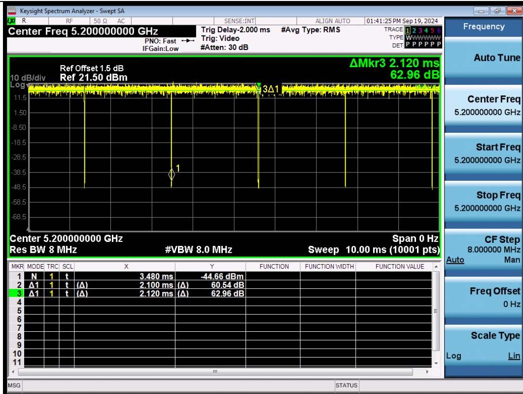
NTNV-11A-Ant1-5200
