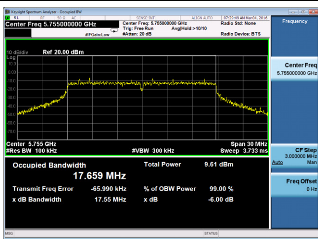
99% & 6dB BW – 20M 5755MHz
