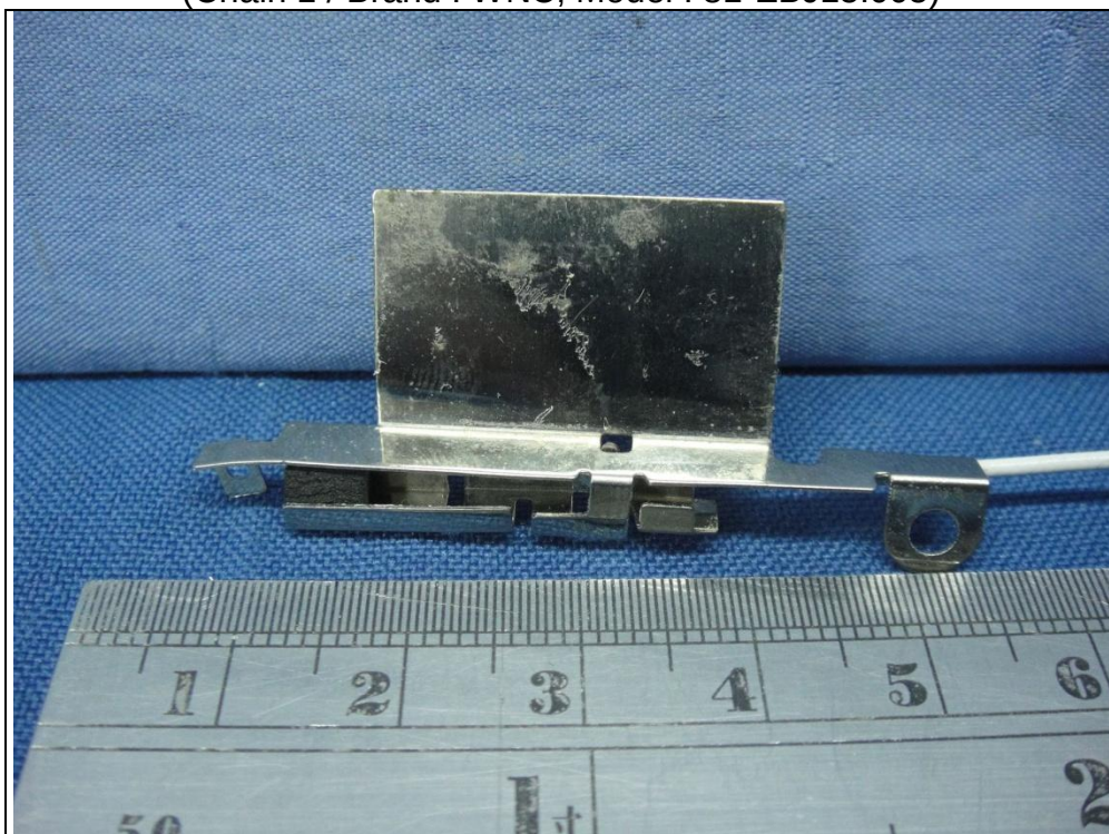
Antenna set 1 (Chain 1 / Brand : WNC, Model : 81-EBJ15.005)
